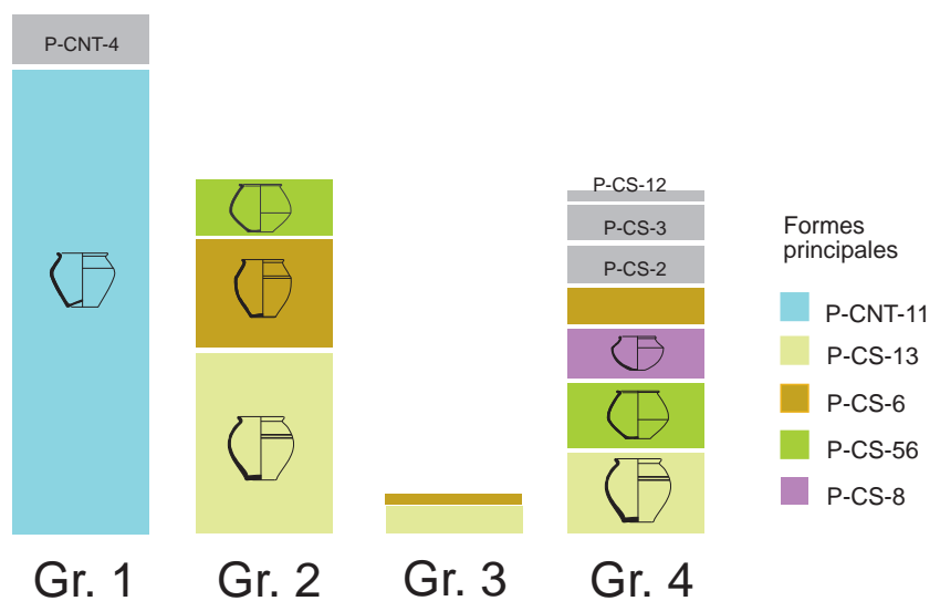
Fig. 141 Graphique de comparaison du répertoire des formes liées aux quatre groupes techniques identifiés. Les référents typologiques dominants sont représentés par des codes couleurs. Pour le détail des quantifications, cf. fig. 140. © R. Delage, Inrap
