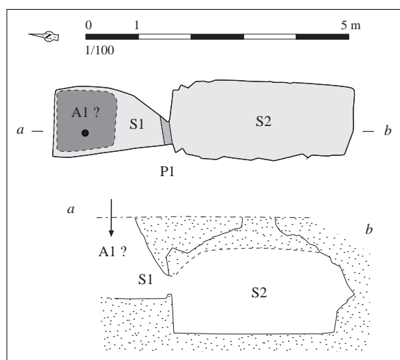
Relevé normalisé de la structure. DAO S. Bossard, d'après Lecornec, 1969, p. 116-117, fig. 4 et 5
