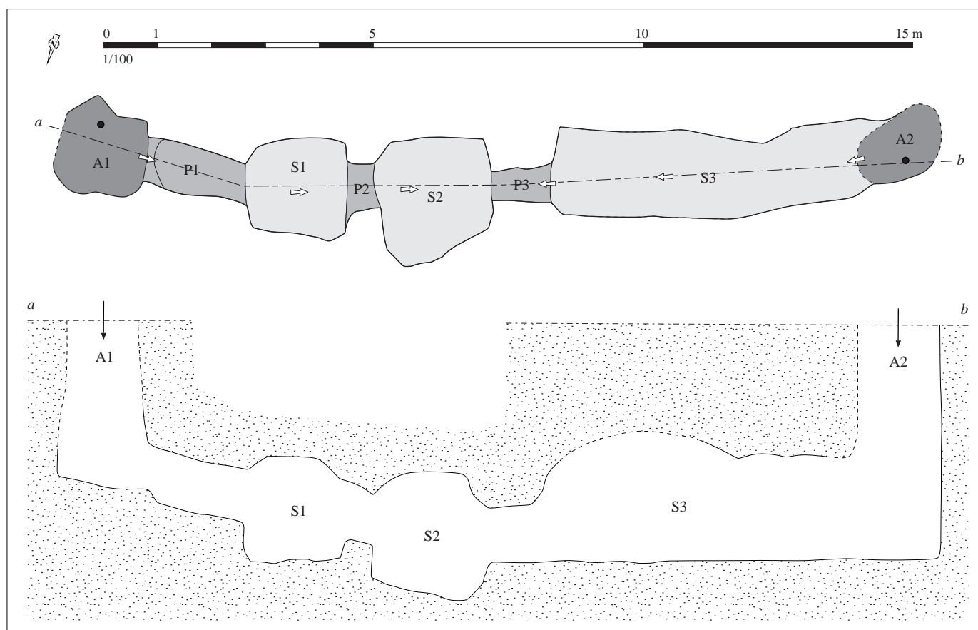
Relevé normalisé de la structure. DAO S. Bossard, d'après Le Roux, Lecerf, 1971, p. 163, fig. 1
