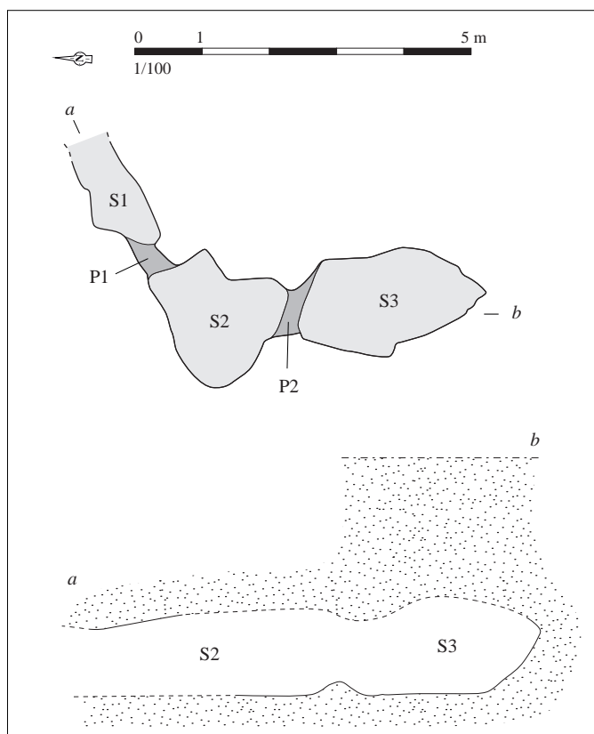
Relevé normalisé de la structure. DAO S. Bossard, d'après Lecerf, 1978, p. 111
