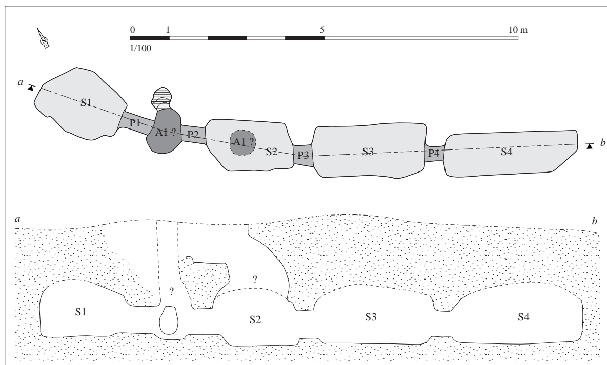
Relevé normalisé de la structure. DAO S. Bossard, d'après Lecornec, 1978, p. 124
