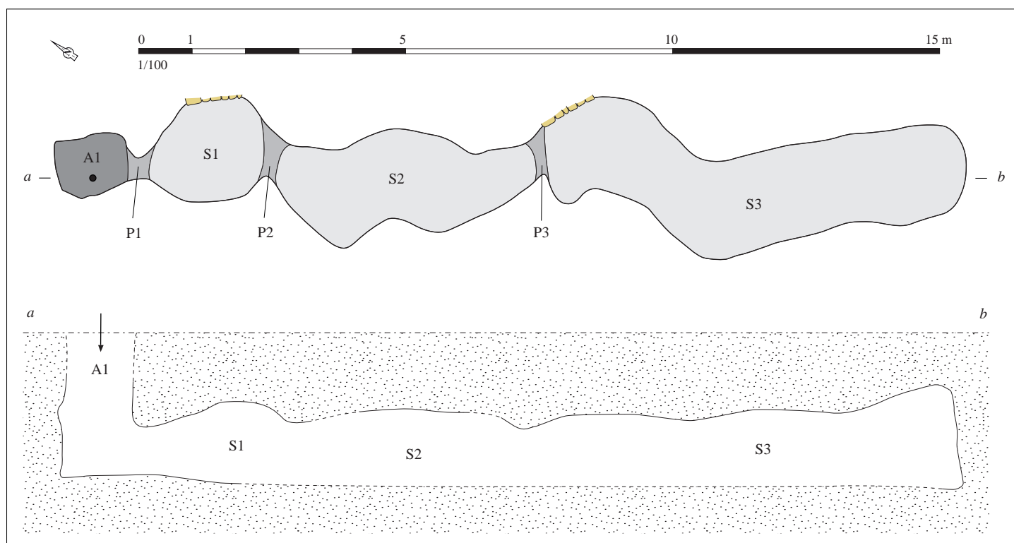
Relevé normalisé de la structure. DAO S. Bossard, d'après Le Brozec, 1991, p. 5
