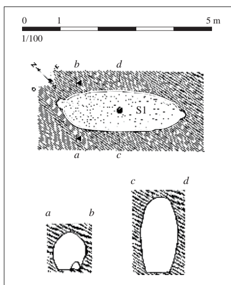
Relevé normalisé de la structure. D'après Aveneau de la Grancière, 1897, fig. 1 à 4
