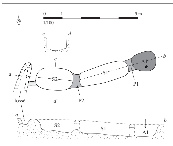
Relevé normalisé de la structure. DAO S. Bossard, d'après Hinguant, 2002, fig. 9
