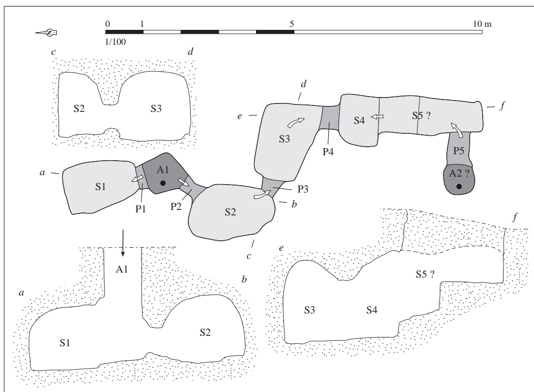
Relevé normalisé de la structure. DAO S. Bossard, d'après Tanguy, 2000, p. 155, fig. 10
