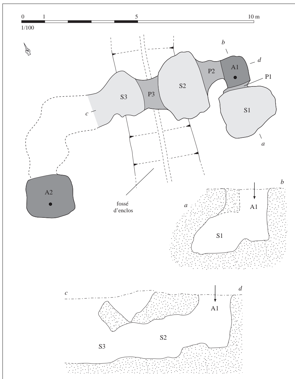
Relevé normalisé de la structure. DAO S. Bossard, d'après Menez, 2009, p. 125, fig. 115
