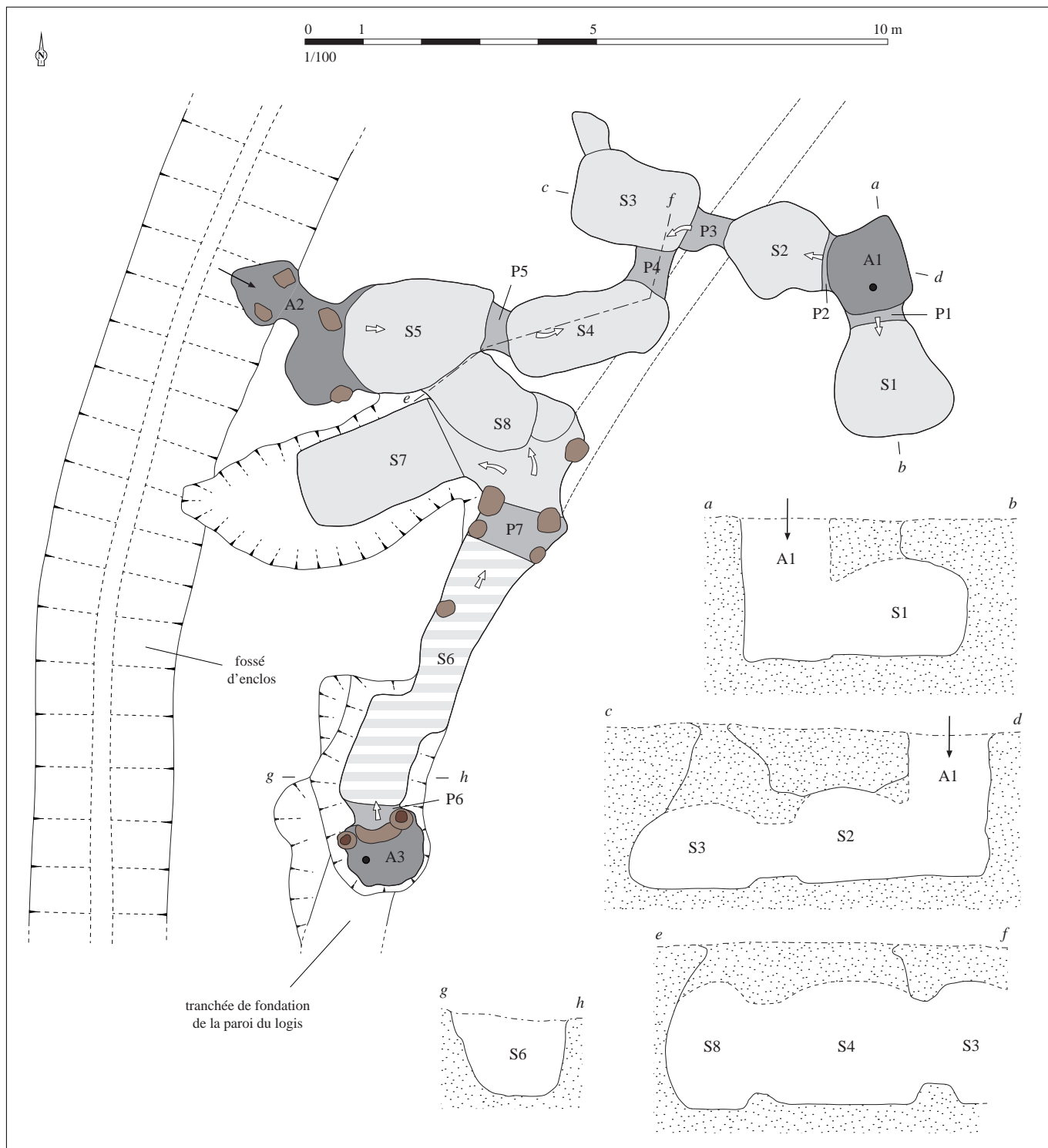
Relevé normalisé de la structure. DAO S. Bossard, d'après Menez, 2009, p. 47, fig. 39
