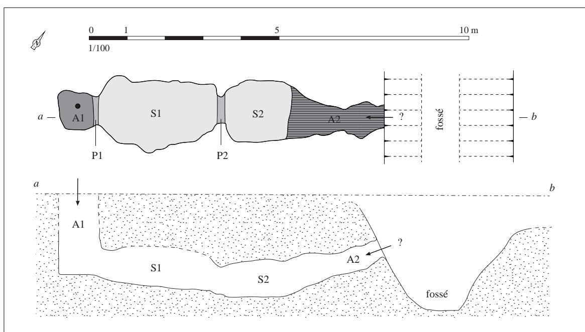
Relevé normalisé de la structure. DAO S. Bossard, d'après Le Goffic et al., 1985, p. 512, fig. 2
