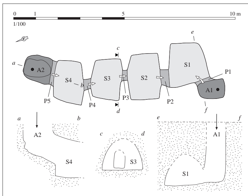
Relevé normalisé de la structure. DAO S. Bossard, d'après Le Roux, 1967, fig. 1 p. 129
