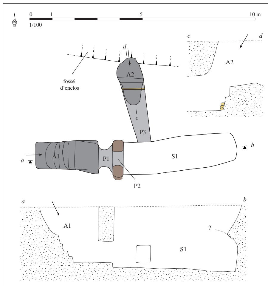
Relevé normalisé de la structure. DAO S. Bossard, d'après Carpentier et al., 2002, p. 46, fig. 9
