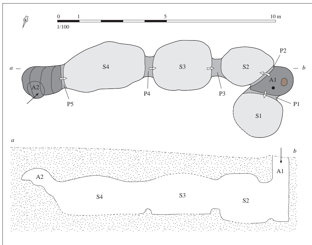
Relevé normalisé de la structure. DAO S. Bossard, d'après Le Goffic, 1984, fig. 1
