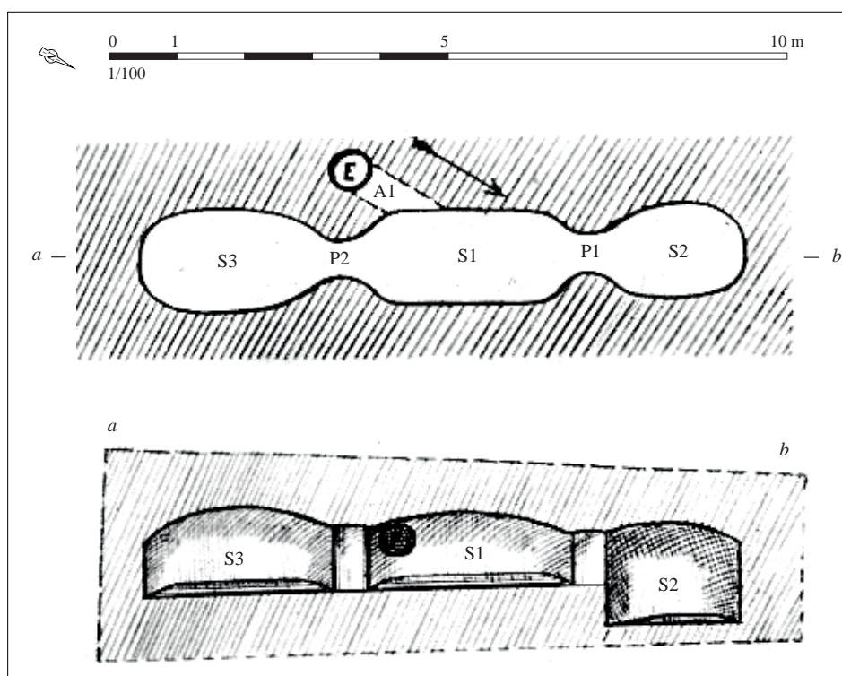
Relevé normalisé de la structure. DAO S. Bossard, d'après Châtellier, 1907, p. 330, pl. XXI
