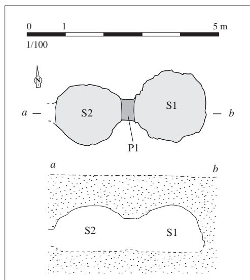
Relevé normalisé de la structure. DAO S. Bossard, d'après Le Goffic, 2002, p. 28, fig. 10
