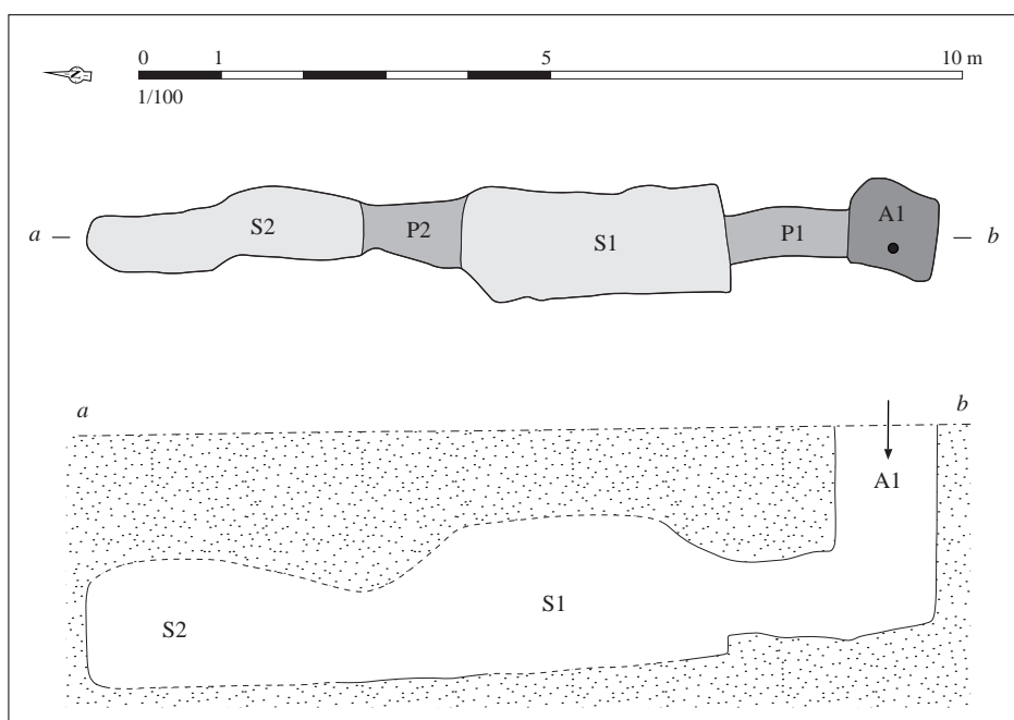
Relevé normalisé de la structure. DAO S. Bossard, d'après Le Roux, 1969, p. 86, fig. 1
