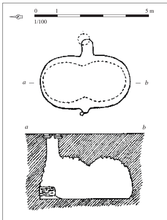
Plan et profil de la structure. D'après Marseille, 1922
