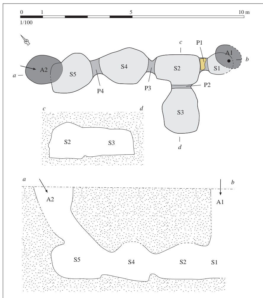
Relevé normalisé de la structure. DAO S. Bossard, d'après Giot et al., 1965, p. 118, fig. 2 et p. 121, fig. 3
