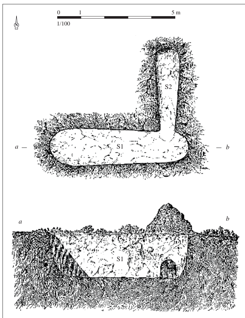
Relevé normalisé de la structure. DAO S. Bossard, d'après la Chênelière, 1876
