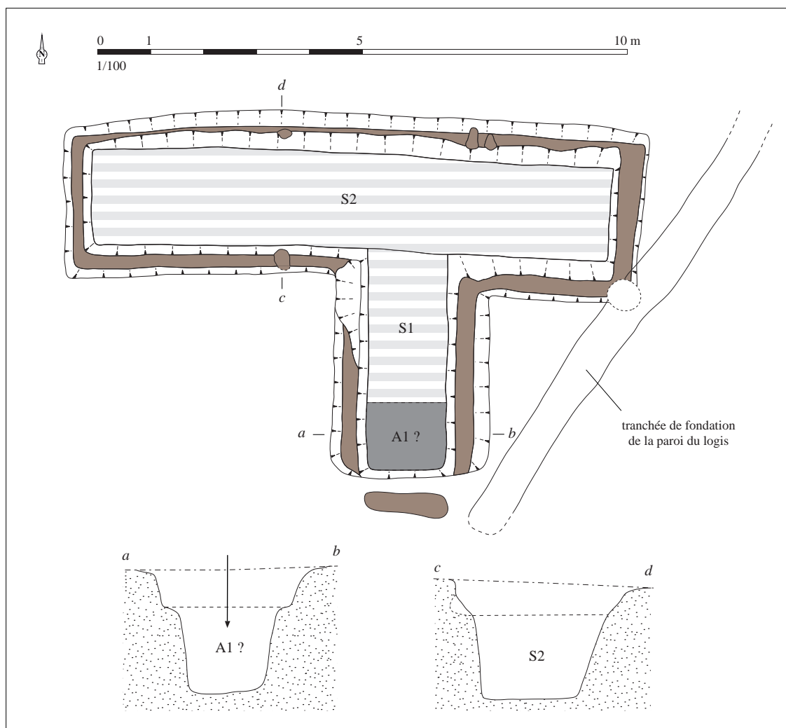
Relevé normalisé de la structure. DAO S. Bossard, d'après Menez, 2009, p. 41, fig. 33
