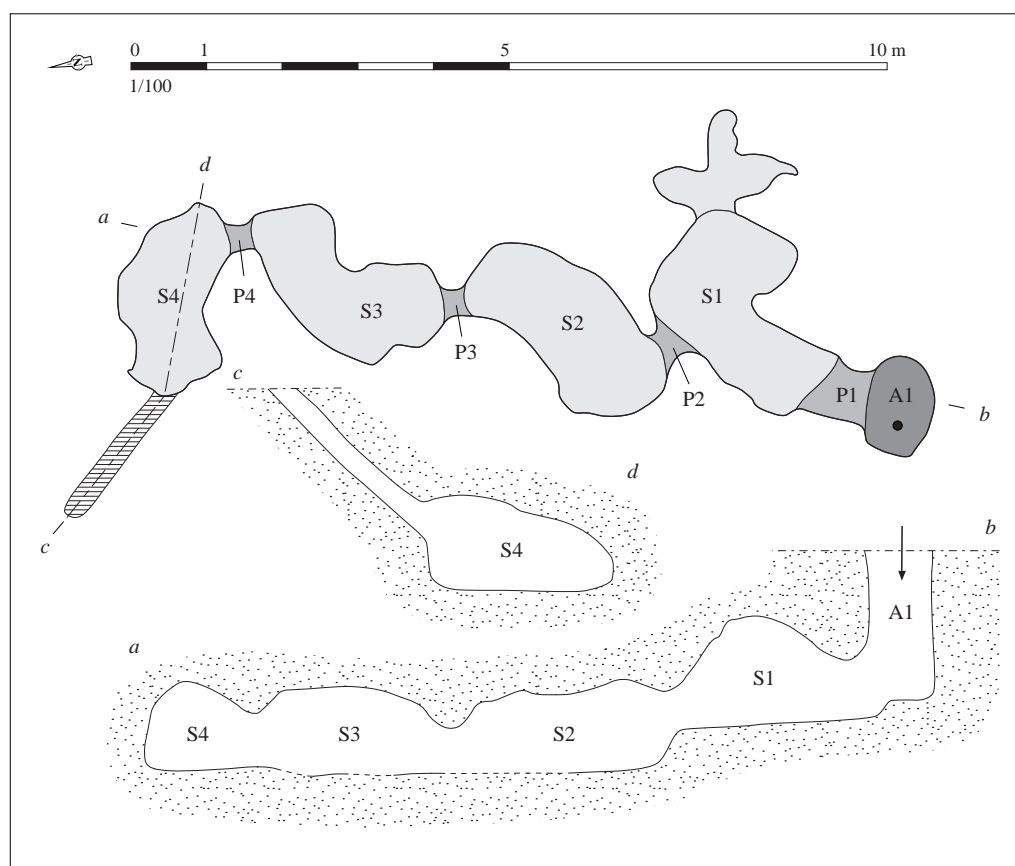
Relevé normalisé de la structure. DAO S. Bossard, d'après Lecerf, 1976, p. 23-24
