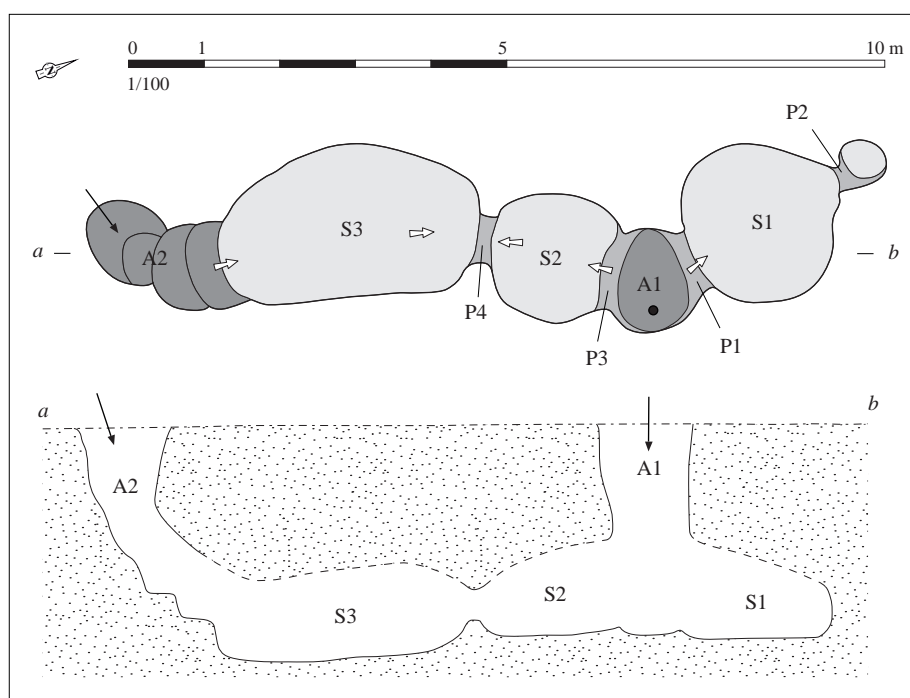
Relevé normalisé de la structure. DAO S. Bossard, d'après Le Goffic, 1987, pl. 2
