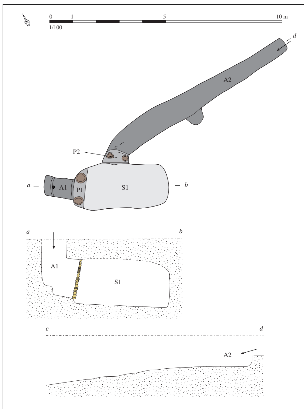
Relevé normalisé de la structure. DAO S. Bossard, d'après Besnard-Vauterin, Guillon, 2009, p. 46, fig. 28
