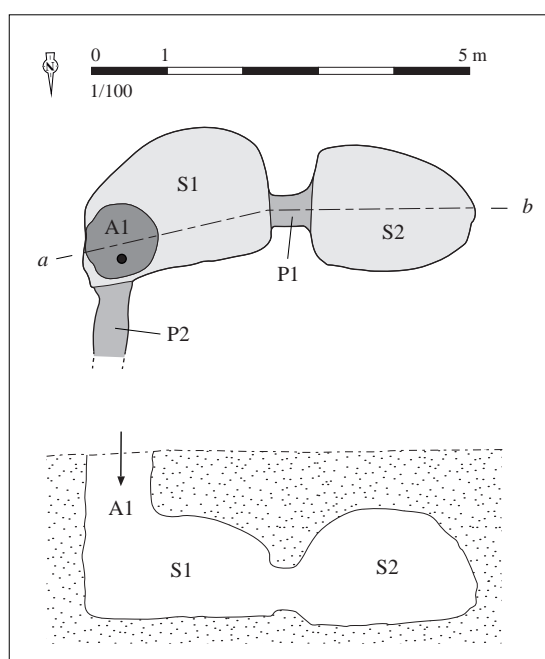
Relevé normalisé de la structure. DAO S. Bossard, d'après Le Goffic, 2001, p. 85, fig. 11
