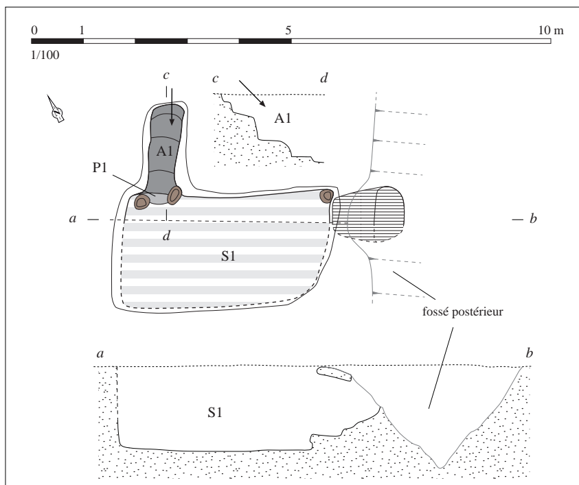
Relevé normalisé de la structure. DAO S. Bossard, d'après Le Goff (dir.), 2002, p. 513, fig. 367
