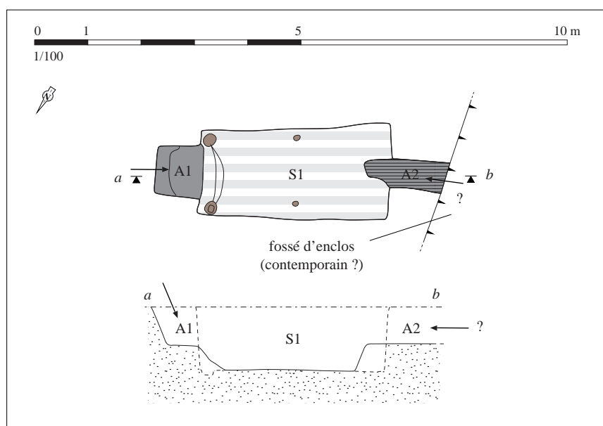
Relevé normalisé de la structure. DAO S. Bossard, d'après Peuchet-Geilenbrügge, 1995, fig. 5
