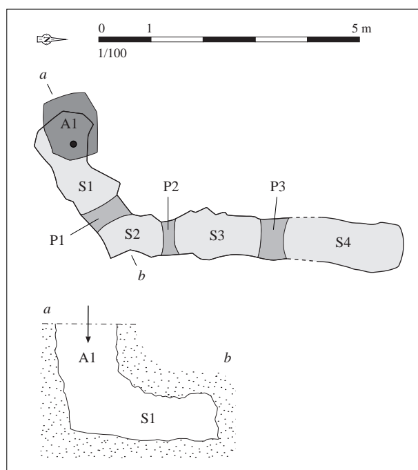
Relevé normalisé de la structure. DAO S. Bossard, d'après Gouletquer, 1983
