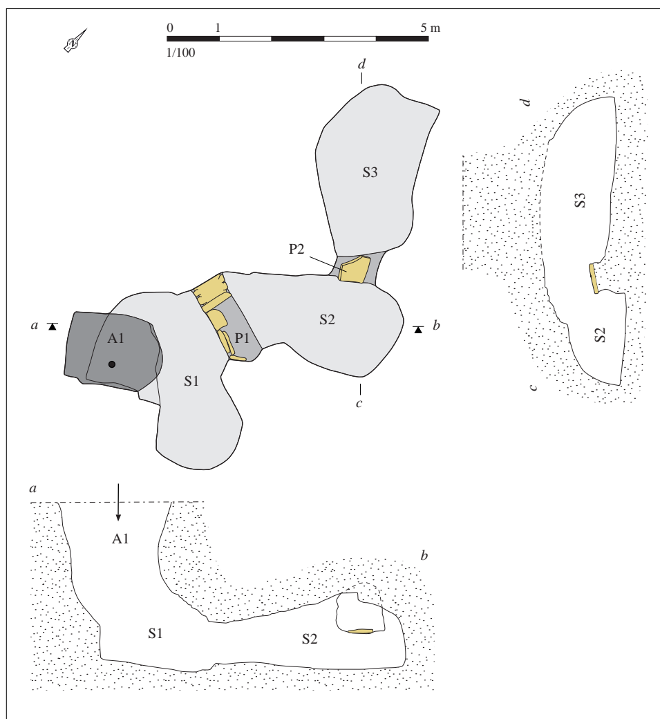
Relevé normalisé de la structure. DAO S. Bossard, d'après Le Goffic M., 1985, fig 3
