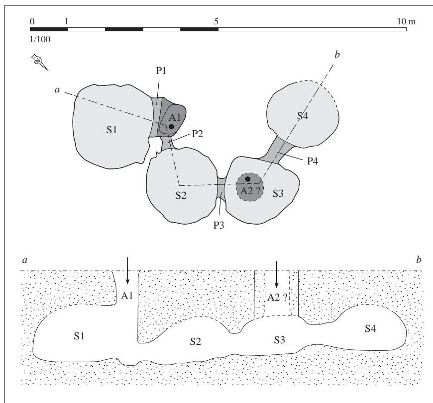
Relevé normalisé de la structure. DAO S. Bossard, d'après M. Guéguen, 1980
