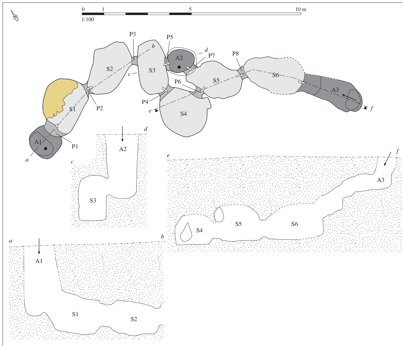
Relevé normalisé de la structure. DAO S. Bossard, d'après Le Goffic, 1997, p. 11, fig. 7
