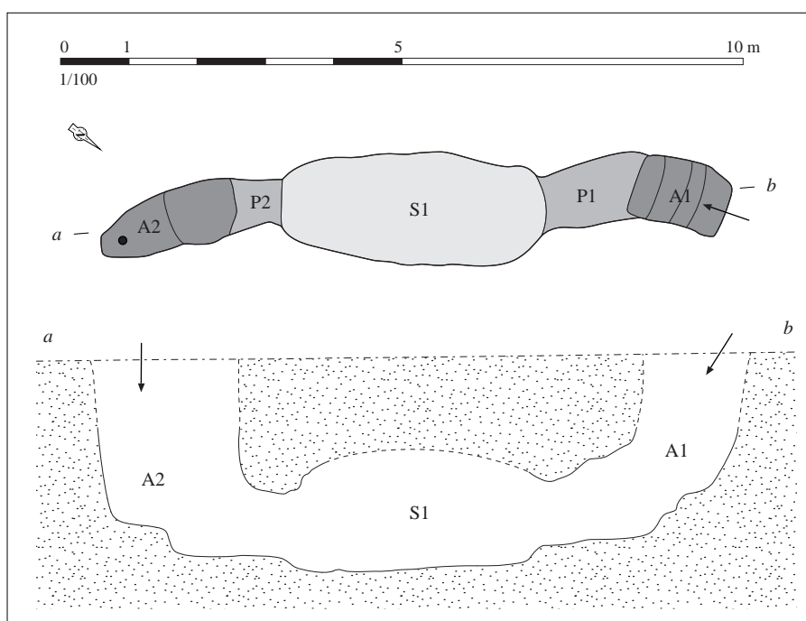
Relevé normalisé de la structure. DAO S. Bossard, d'après Peuchet-Geilenbrügge, 1995, fig. 6
