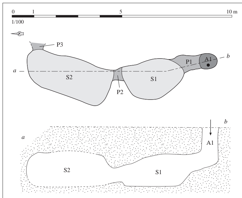
Relevé normalisé de la structure. DAO S. Bossard, d'après Lecerf, 1986
