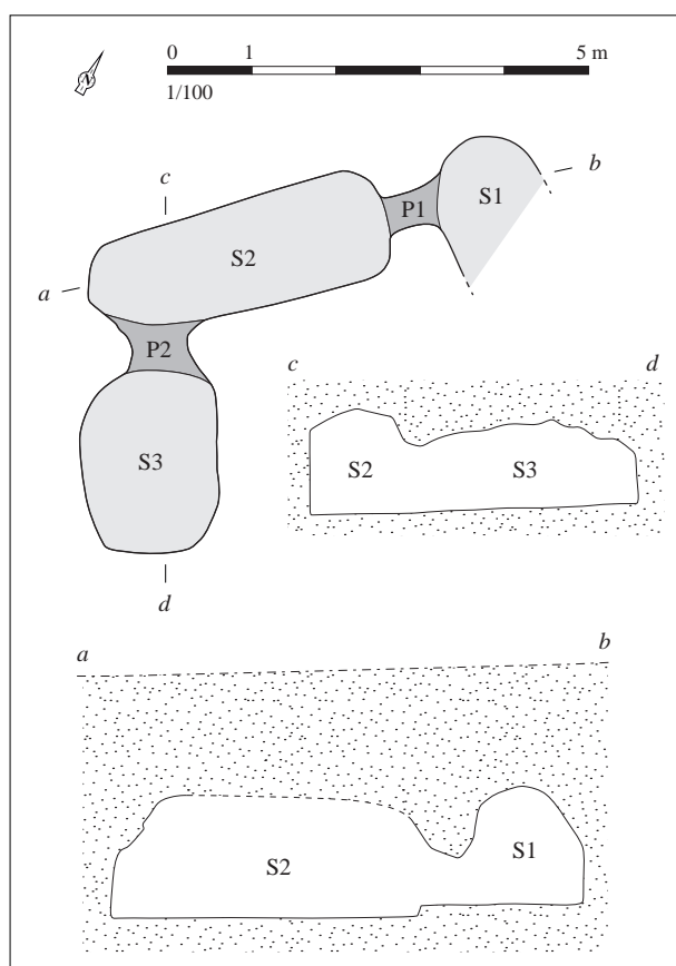
Relevé normalisé de la structure. DAO S. Bossard, d'après Lecornec, 1972, p. 101, fig. 1
