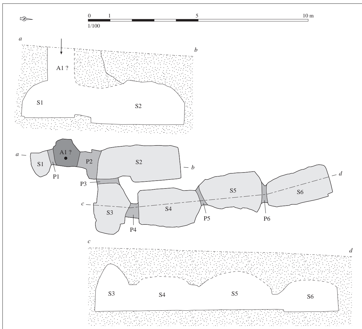
Relevé normalisé de la structure. DAO S. Bossard, d'après Lecornec, 1970, p. 60, fig. 2 et p. 62, fig. 3
