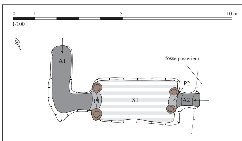
Relevé normalisé de la structure. DAO S. Bossard, d'après Le Goff (dir.), 2002, p. 516, fig. 369
