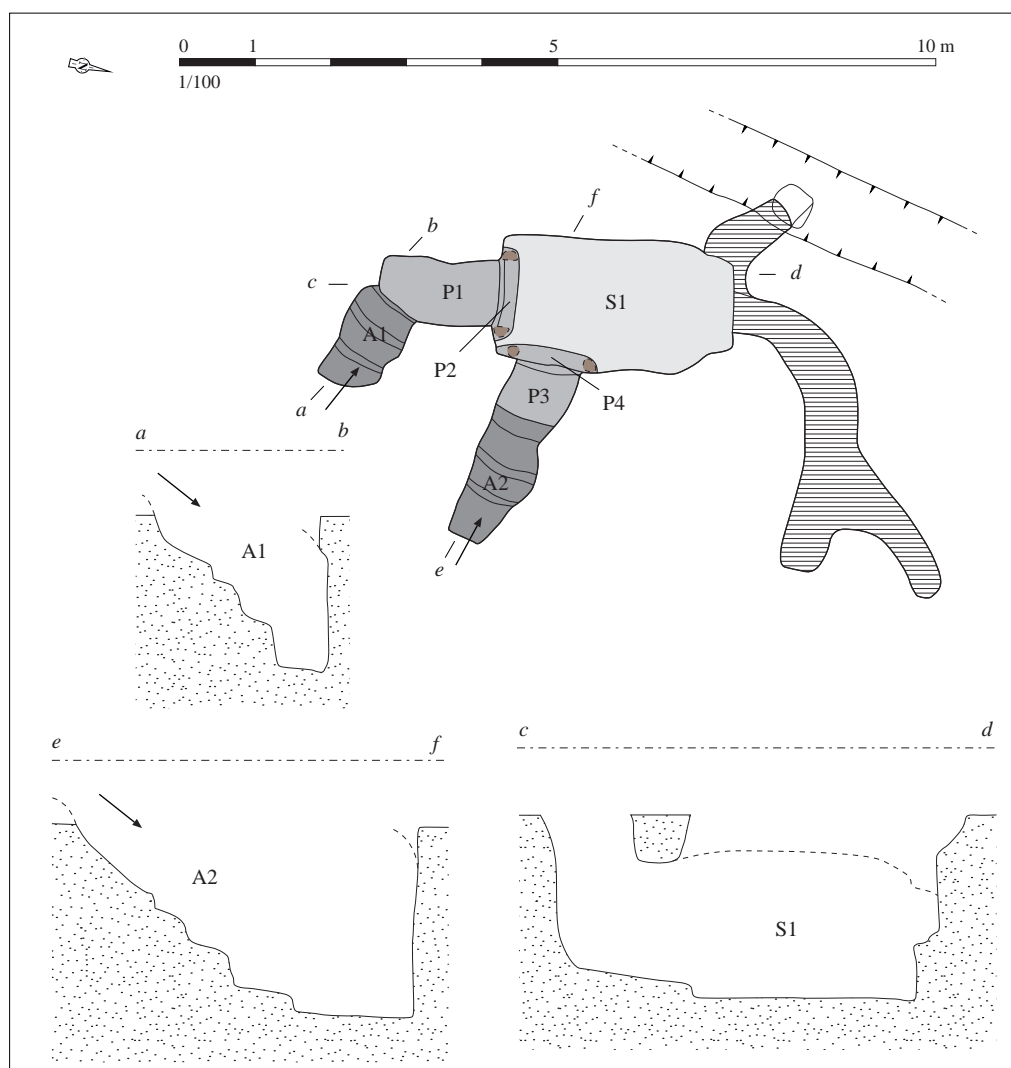
Relevé normalisé de la structure. DAO S. Bossard, d'après Besnard-Vauterin, Guillon, 2009, p. 49, fig. 31
