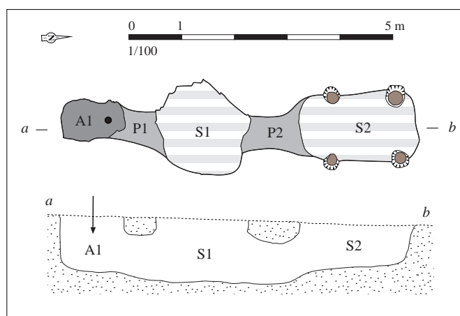
Relevé normalisé de la structure. DAO S. Bossard, d'après Bardel, 1985
