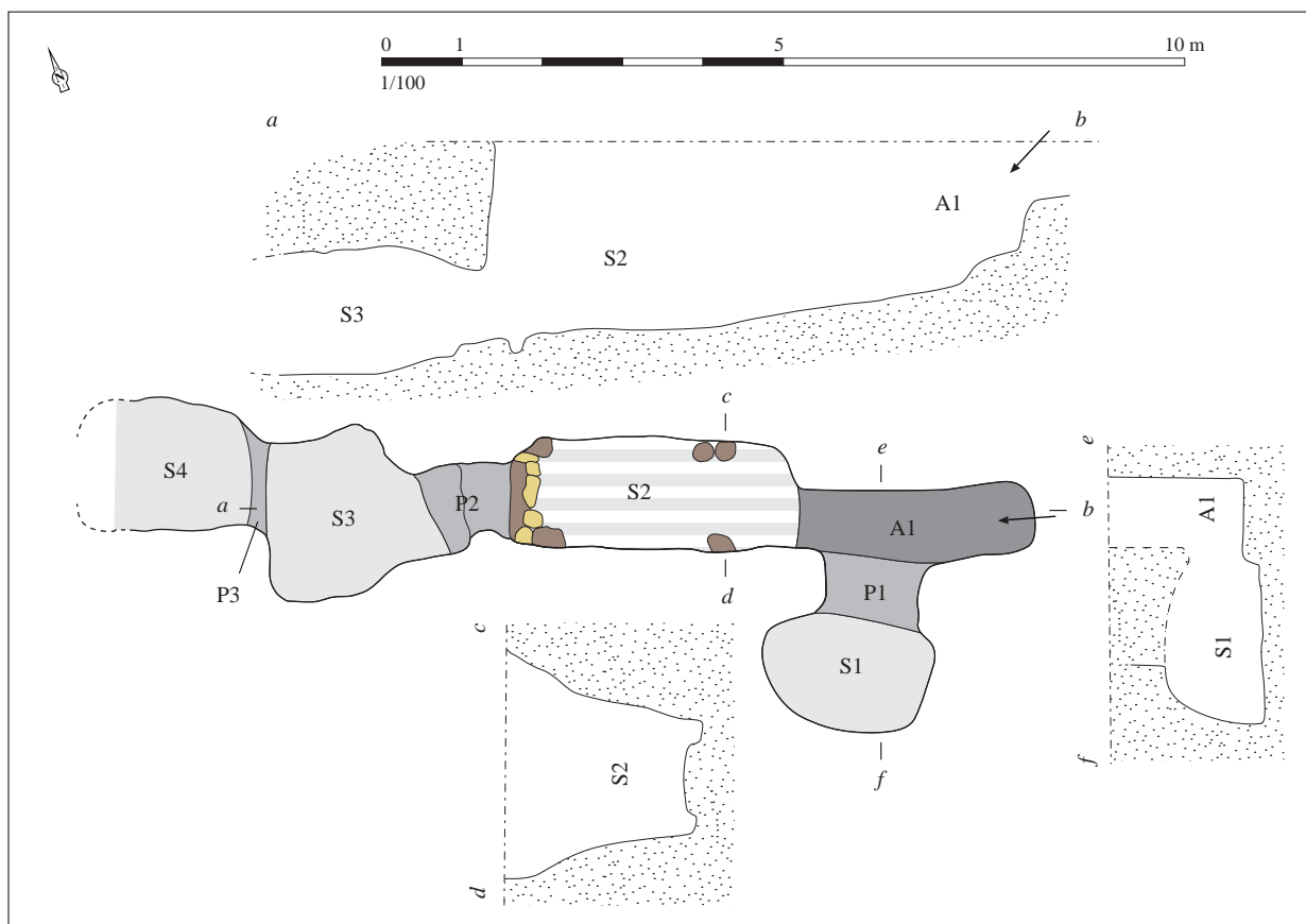
Relevé normalisé de la structure. DAO S. Bossard, d'après Tanguy, 1997, p. 13, fig. 8
