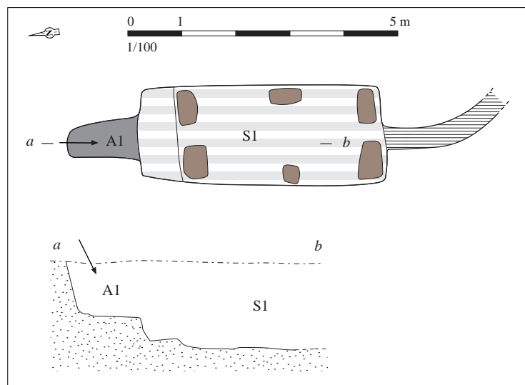
Relevé normalisé de la structure. DAO S. Bossard, d'après Lepaumier (dir.), 2009, p. 43, fig. 18
