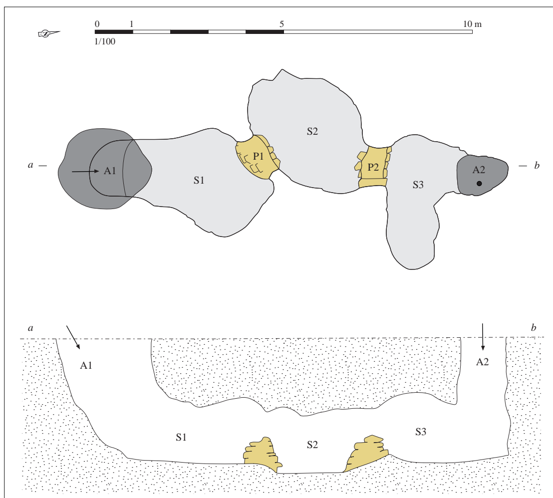
Relevé normalisé de la structure. DAO S. Bossard, d'après Le Goffic, 1984, fig. 1
