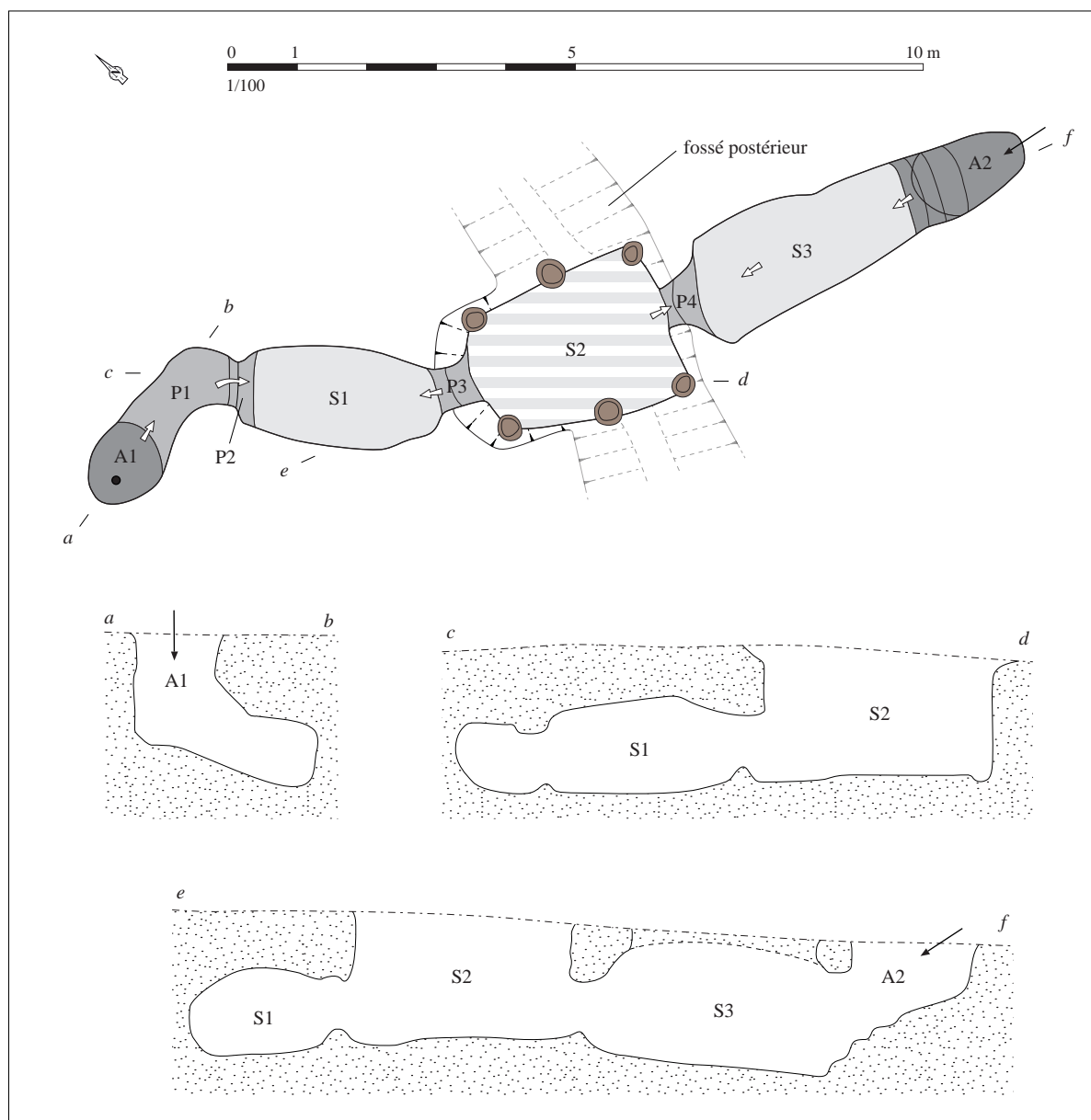
Relevé normalisé de la structure. DAO S. Bossard, d'après Bardel, 1989
