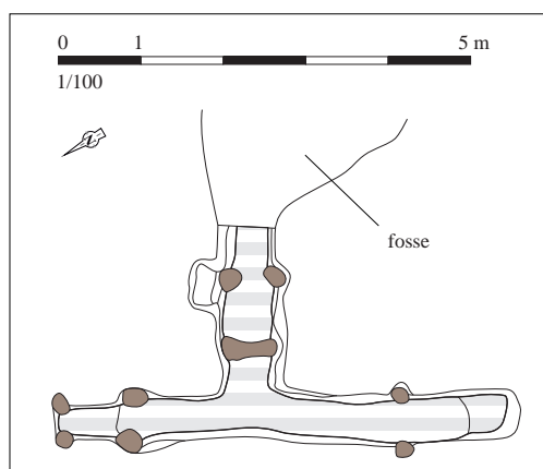
Relevé normalisé de la structure. DAO S. Bossard, d'après Carpentier et al., 2002, p. 44, fig. 8
