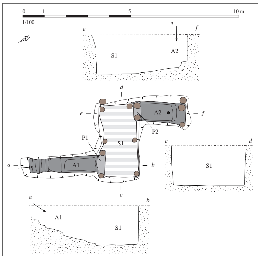
Relevé normalisé de la structure. DAO S. Bossard, d'après Besnard-Vauterin (dir.), 2009, fig. 11
