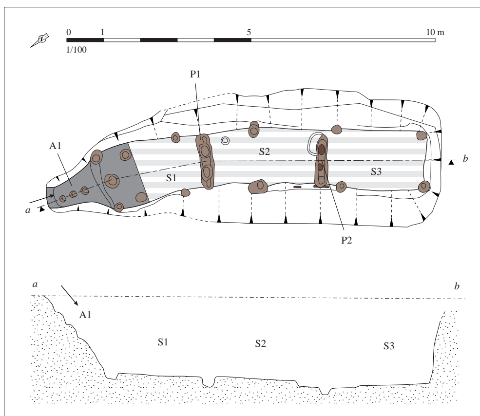
Relevé normalisé de la structure. DAO S. Bossard, d'après Nicolas dir., 2013, p. 80, fig. 50 et p. 82, fig. 55
