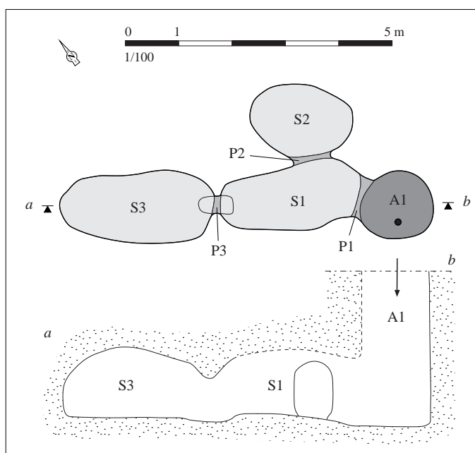
Relevé normalisé de la structure. DAO S. Bossard, d'après Giot, Lecerf, 1971, p. 151, fig. 1
