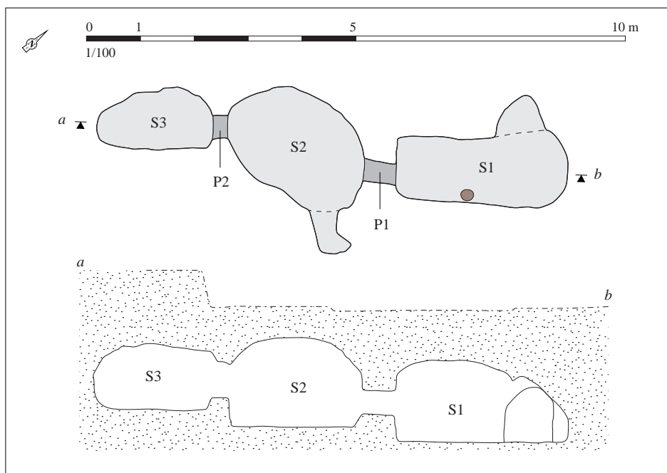
Relevé normalisé de la structure. DAO S. Bossard, d'après Lecornec, 1997, p. 18, fig. 2
