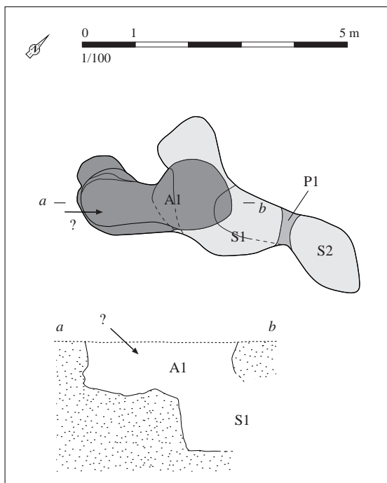
Relevé normalisé de la structure. DAO S. Bossard, d'après D. Etienne
