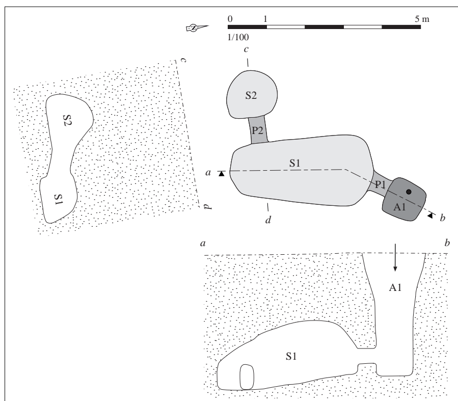
Relevé normalisé de la structure. DAO S. Bossard, d'après anonyme, 1982
