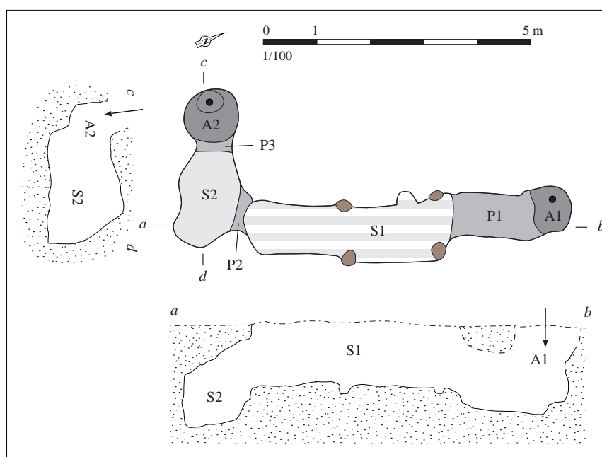
Relevé normalisé de la structure. DAO S. Bossard, d'après Tanguy et al., 2000, p. 149, fig. 5
