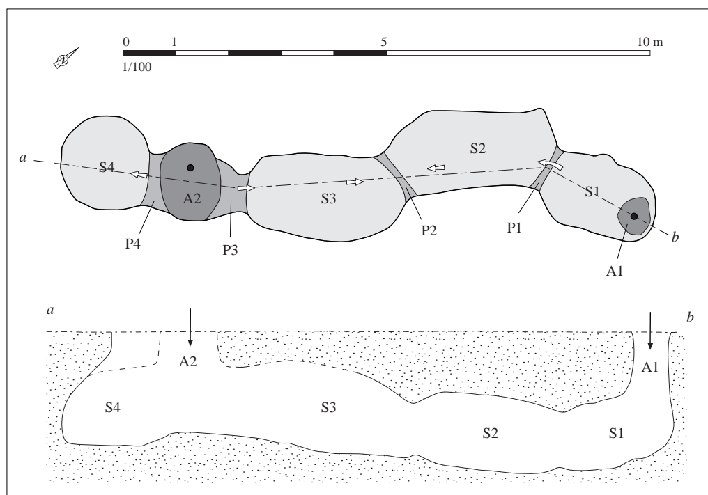
Relevé normalisé de la structure. DAO S. Bossard, d'après Giot, Le Roux, 1965, p. 98, fig. 2
