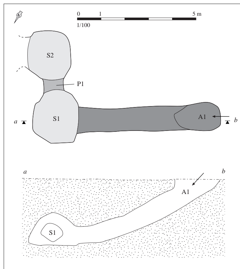
Relevé normalisé de la structure. DAO S. Bossard, d'après la documentation du SRA Bretagne
