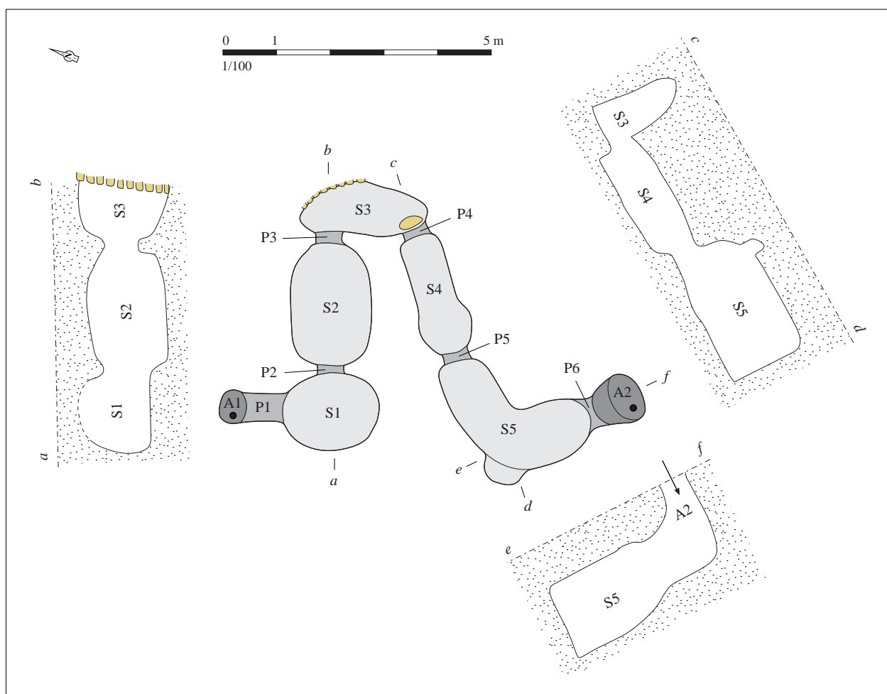
Relevé normalisé de la structure. DAO S. Bossard, d'après Giot et al., 1970, p. 77, fig. 2
