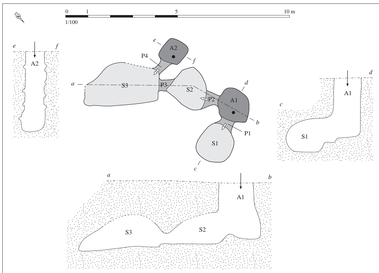
Relevé normalisé de la structure. DAO S. Bossard, d'après Le Roux, Colombel, 1978, p. 48
