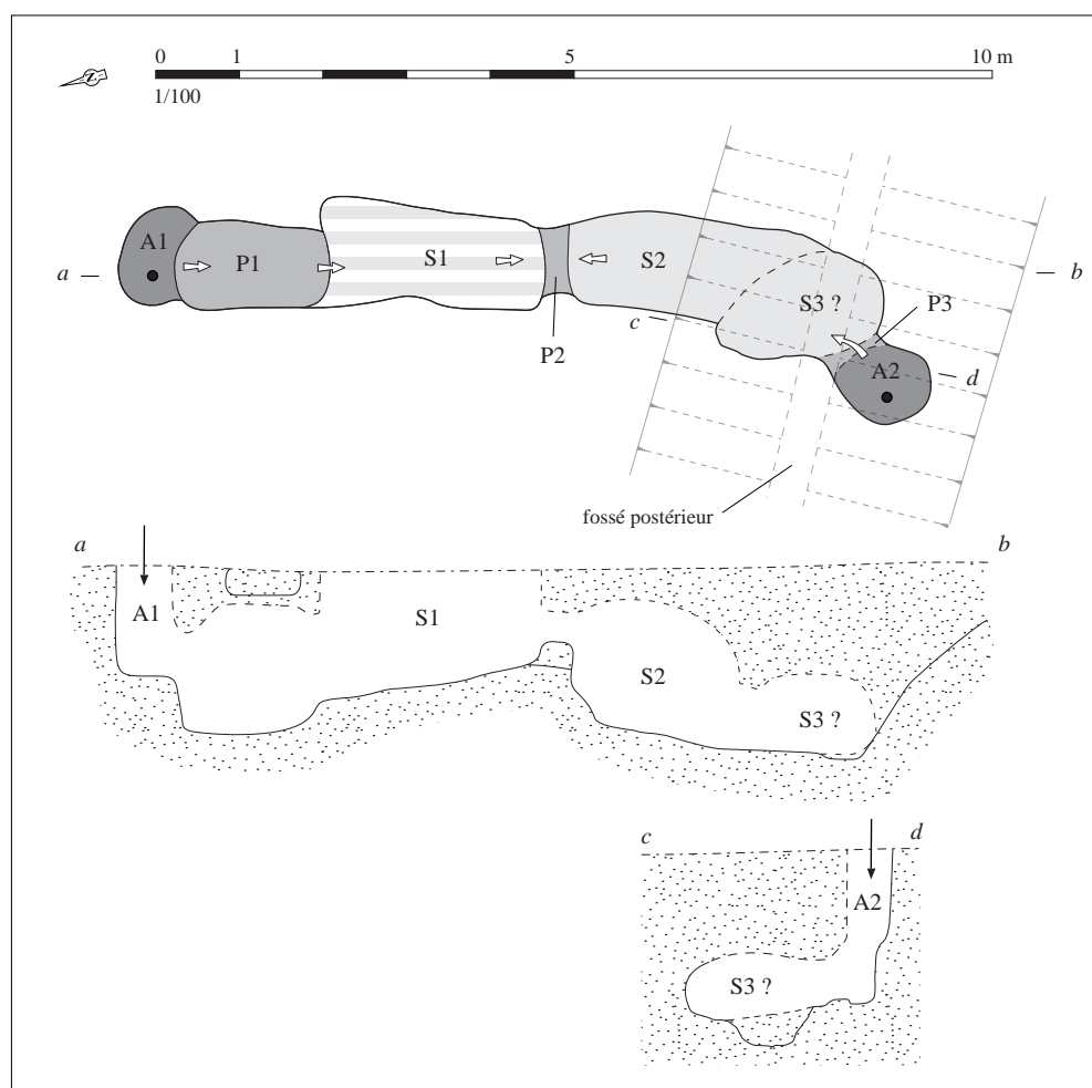
Relevé normalisé de la structure. DAO S. Bossard, d'après Tanguy, 2006, p. 13, fig. 10
