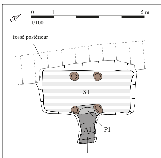
Relevé normalisé de la structure. DAO S. Bossard, d'après Le Goff (dir.), 2002, p. 503, fig. 362
