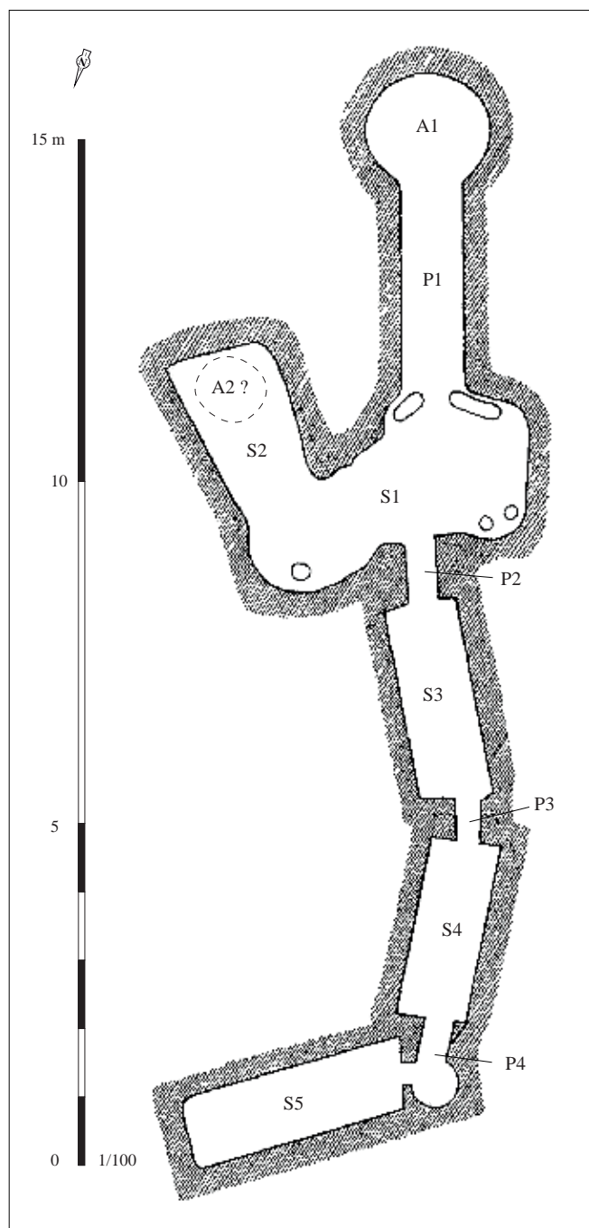
Relevé normalisé de la structure. D'après Bélizal, 1889, pl. I
