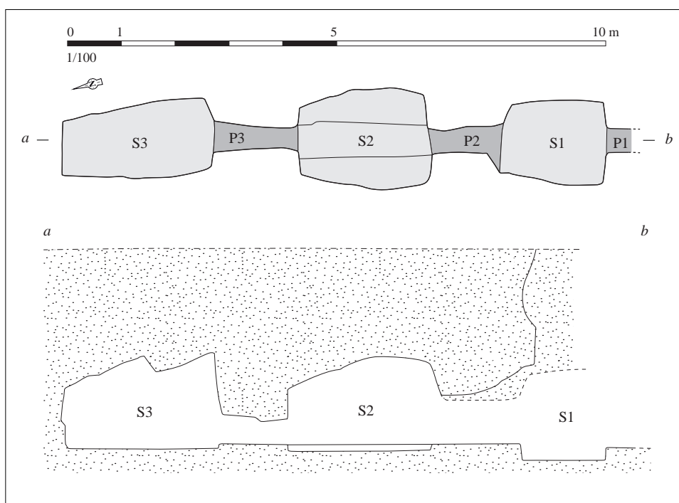
Relevé normalisé de la structure. DAO S. Bossard, d'après Lecornec, 1969, p. 110, fig. 1
