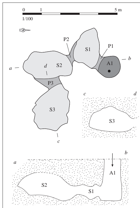
Relevé normalisé de la structure. DAO S. Bossard, d'après Lecerf, 1978, p. 100
