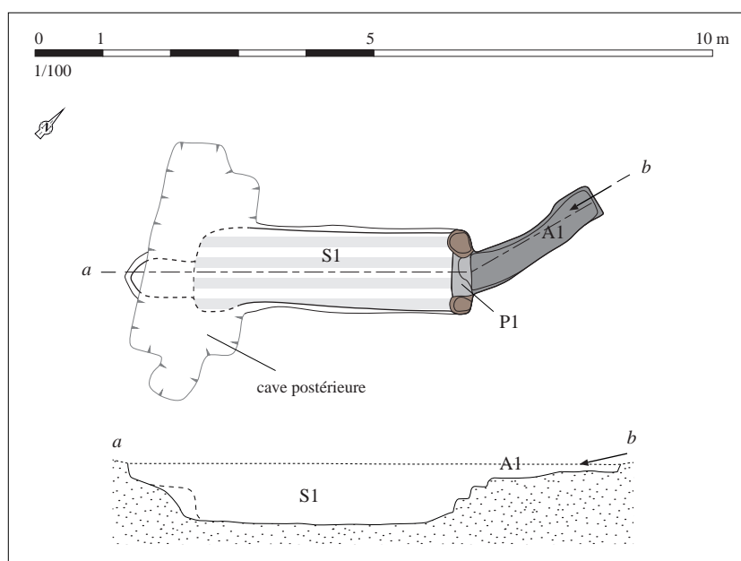
Relevé normalisé de la structure. DAO S. Bossard, d'après Le Goff (dir.), 2002, p. 265, fig. 182
