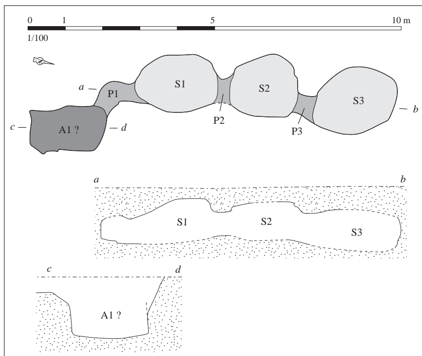
Relevé normalisé de la structure. DAO S. Bossard, d'après Bardel, 1993
