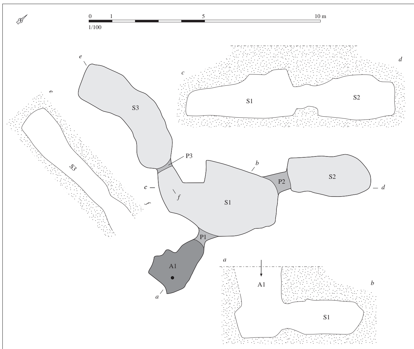
Relevé normalisé de la structure. DAO S. Bossard, d'après Gouletquer, 1969, p. 38, fig. 1
