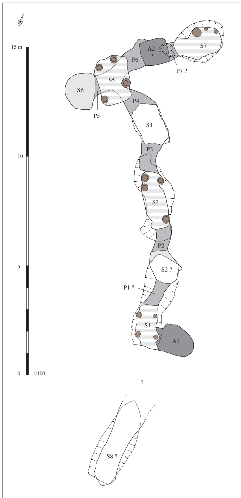
Relevé normalisé de la structure. DAO S. Bossard, d'après Bardel, 1988
