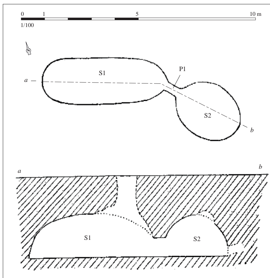
Relevé de la structure. DAO S. Bossard, d'après Marseille, 1916, p. 25
