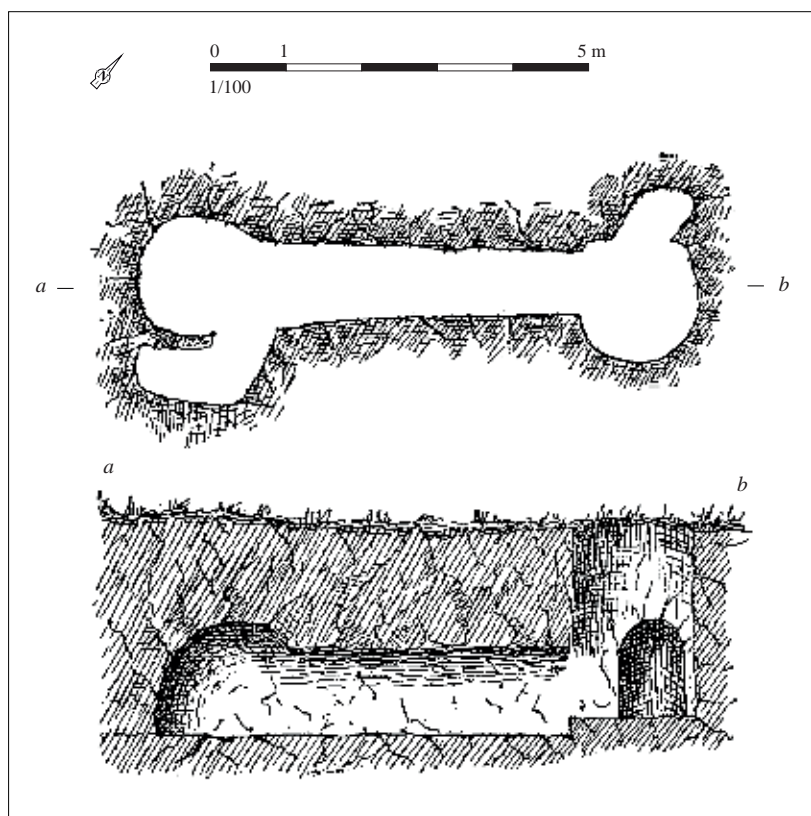
Relevé de la structure. DAO S. Bossard, d'après Anne Duportal, 1901, p. 21, fig. 1 et 2
