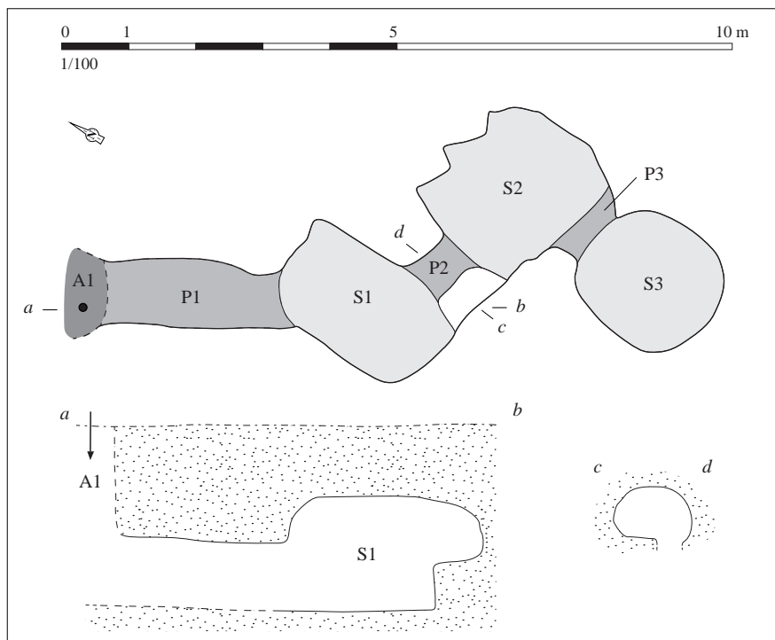
Relevé normalisé de la structure. DAO S. Bossard, d'après Bar- del, 1982
