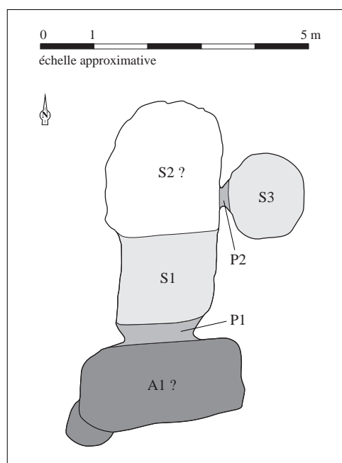
Relevé normalisé de la structure. DAO S. Bossard, d'après Nivart, 1980
