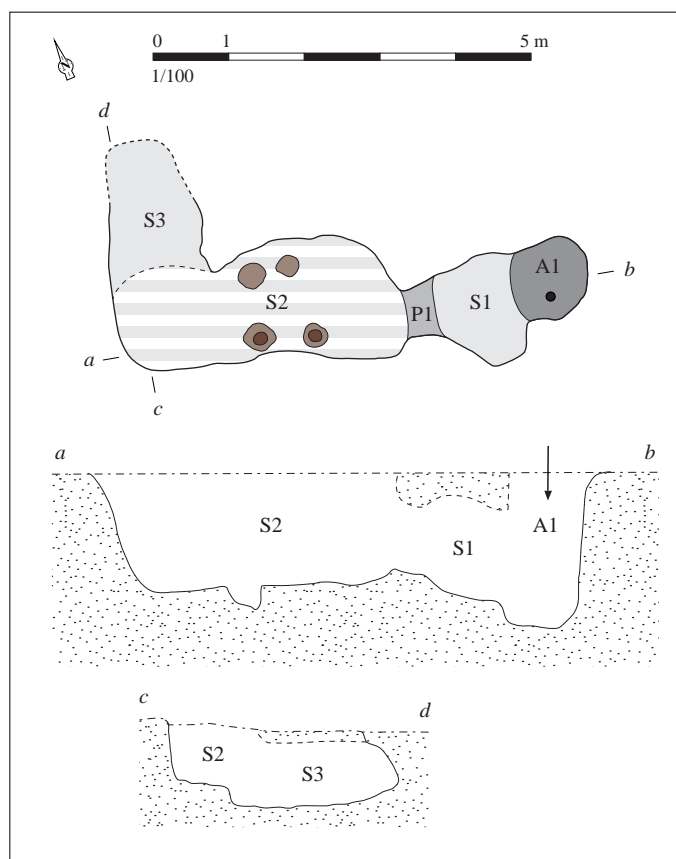
Relevé normalisé de la structure. DAO S. Bossard, d'après Menez, 2009, p. 122, fig. 112
