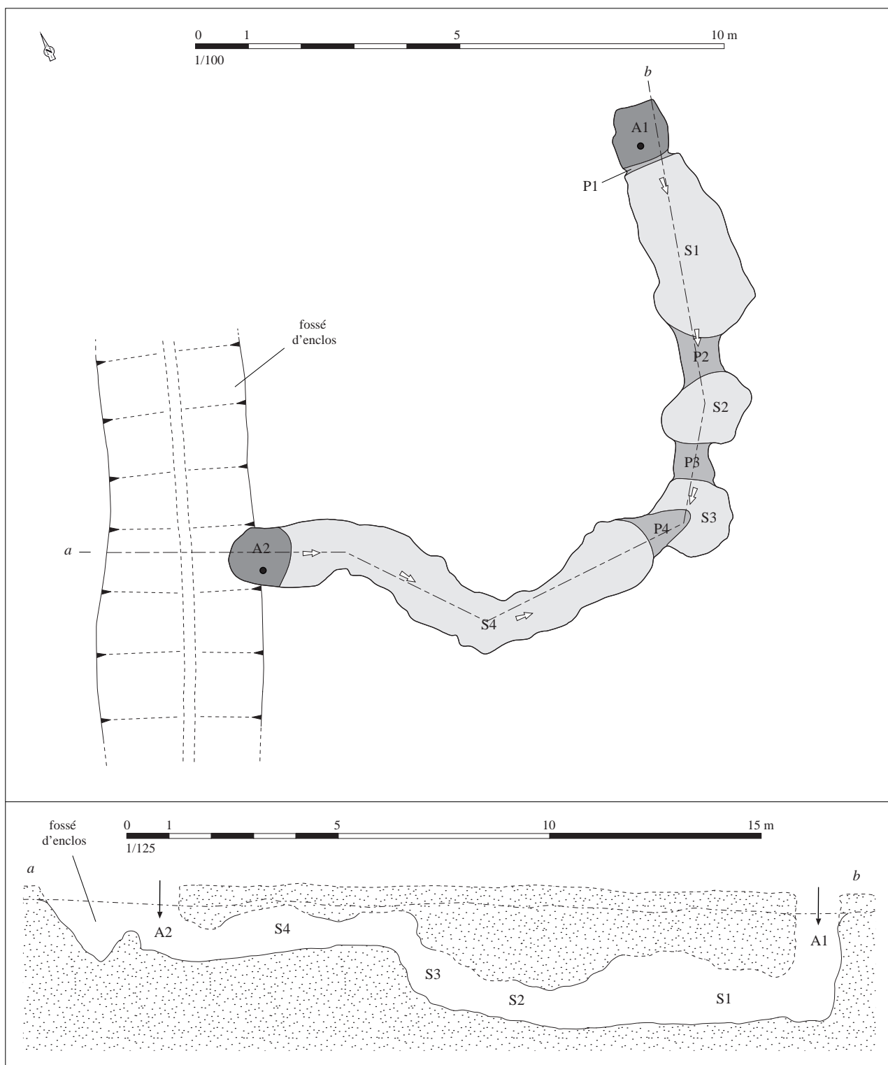
Relevé normalisé de la structure. DAO S. Bossard, d'après Menez, 2009, p. 123-124, fig. 113 et 114
