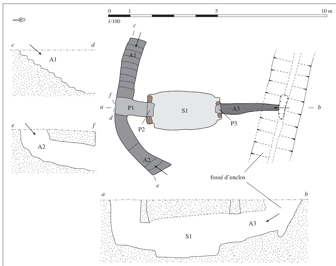
Relevé normalisé de la structure. DAO S. Bossard, d'après Marcigny, 1995, p. 67, fig. 37
