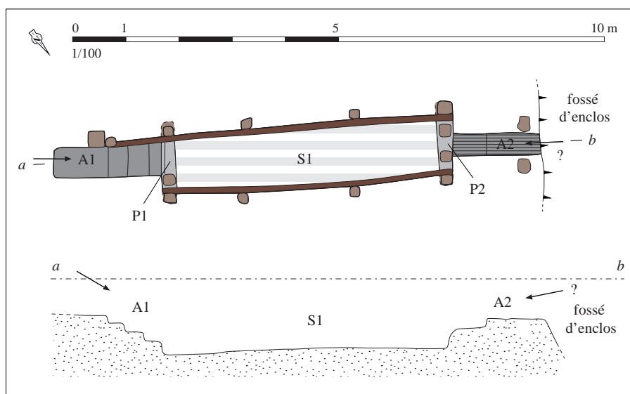
Relevé normalisé de la structure. DAO S. Bossard, d'après Marcigny et al., 2004, p. 78, fig. 15
