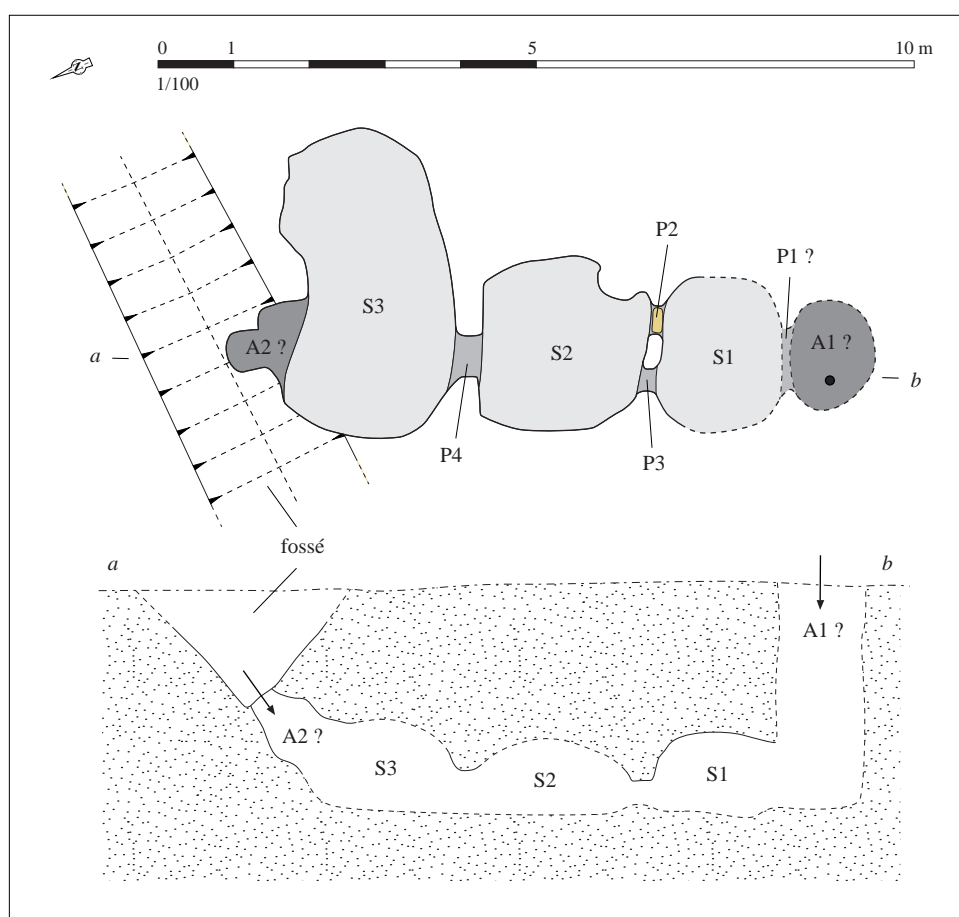
Relevé normalisé de la structure. DAO S. Bossard, d'après Le Goffic, 2000, p. 39, fig. 12
