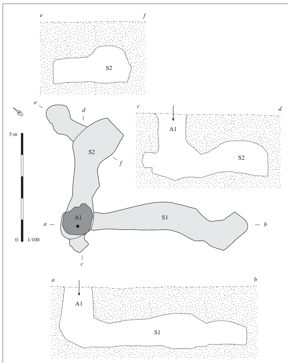
Relevé normalisé de la structure. DAO S. Bossard, d'après Menez (dir.), 1996, fig. 60 p. 63
