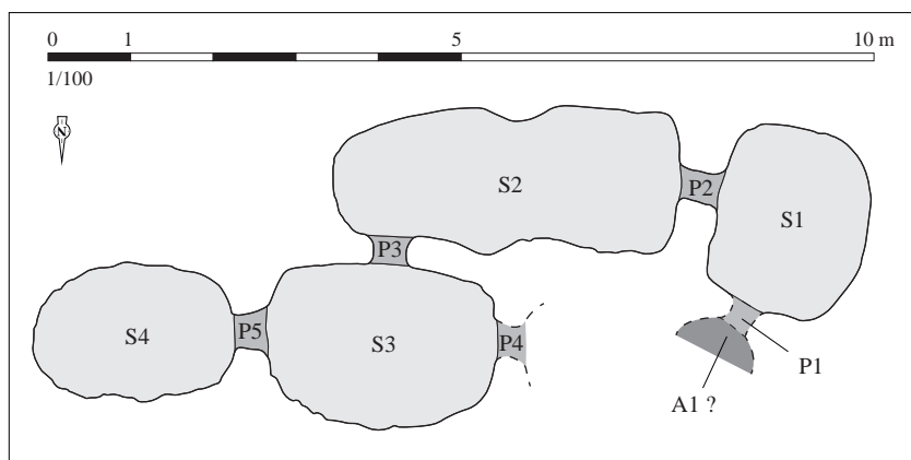
Relevé normalisé de la structure. DAO S. Bossard, d'après Le Goffic, 2010, p. 11, fig. 2
