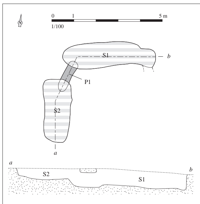
Relevé normalisé de la structure. DAO S. Bossard, d'après Bardel, 1986
