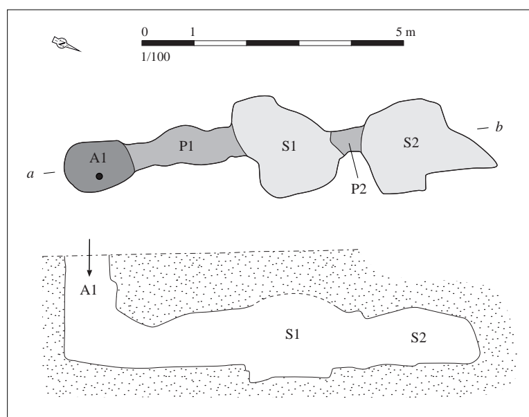
Relevé normalisé de la structure. DAO S. Bossard, d'après Gouletquer, 1969, p. 51, fig. 1
