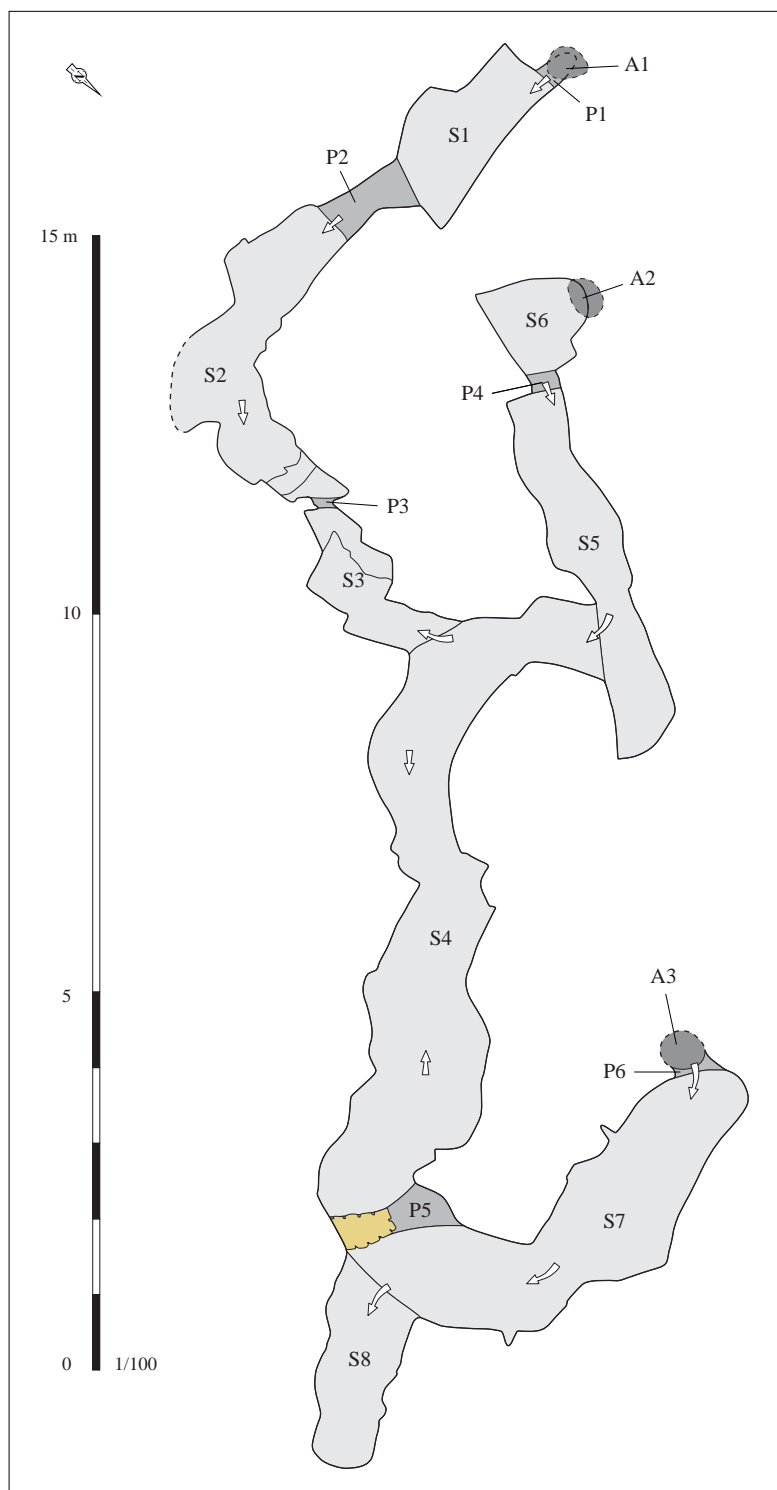
Relevé normalisé de la structure. DAO S. Bossard, d'après Le Roux, Lecerf, 1973, p. 80-81, fig. 1 et 1 bis
