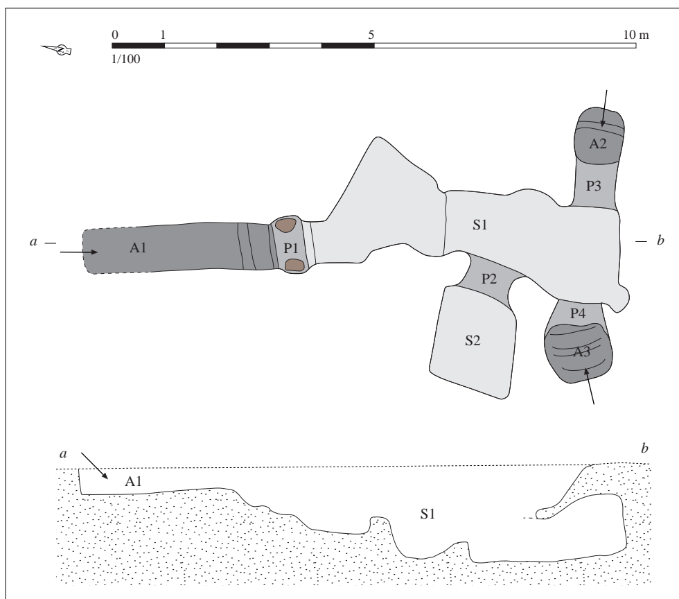
Relevé normalisé de la structure. DAO S. Bossard, d'après Peuchet-Geilenbrügge, 1995, fig. 17
