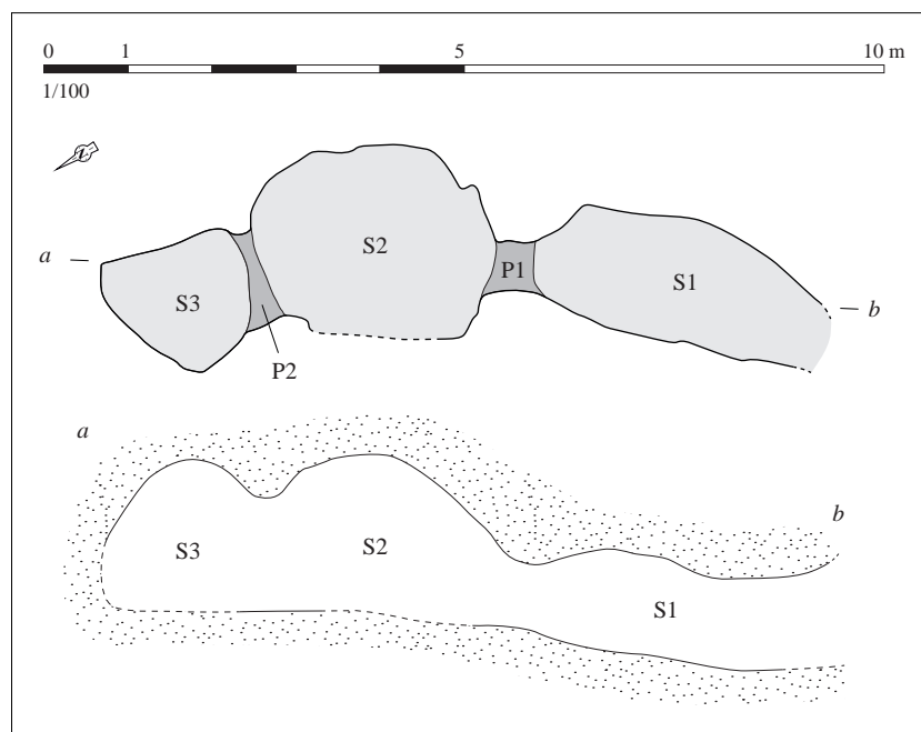
Relevé normalisé de la structure. DAO S. Bossard, d'après Lecerf, 1978, p. 117
