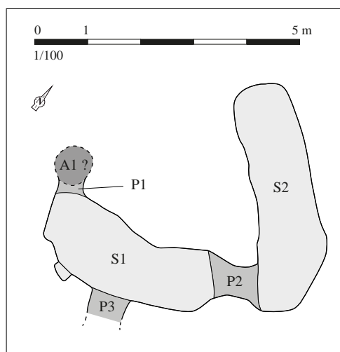
Relevé normalisé de la structure. DAO S. Bossard, d'après la documentation du SRA Bretagne
