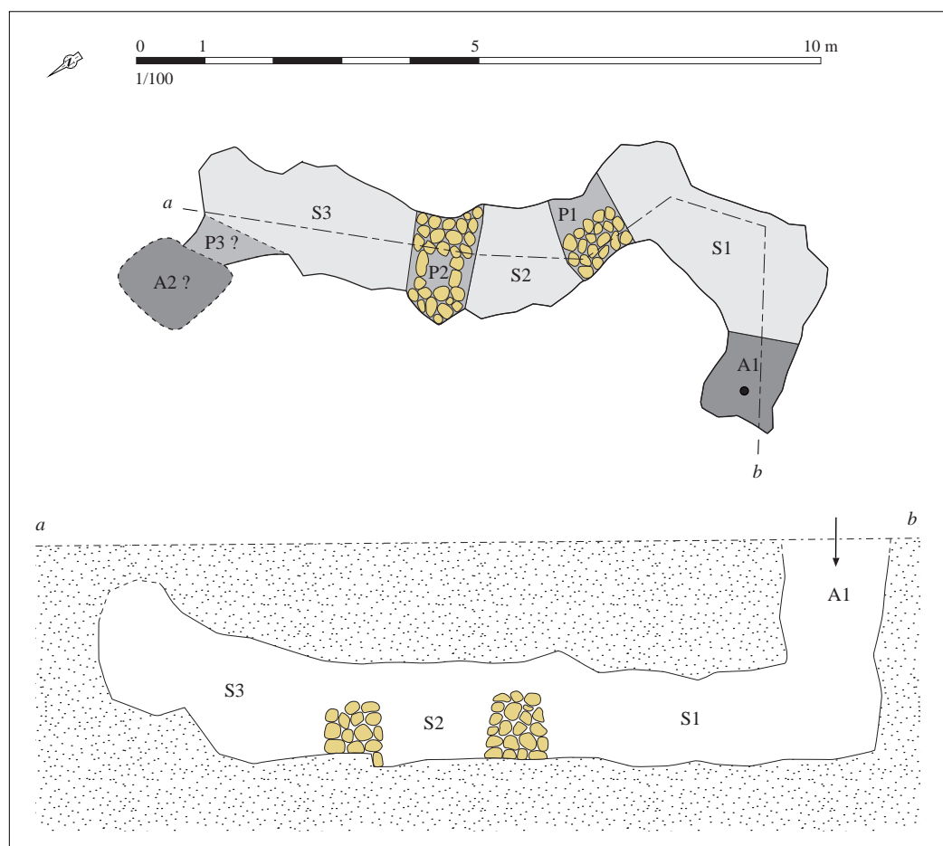
Relevé normalisé de la structure. DAO S. Bossard, d'après Guyader, 1969, p. 64-65, fig. 1 et 2
