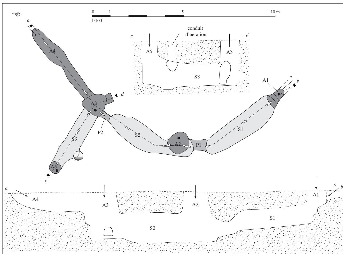
Relevé normalisé de la structure. DAO S. Bossard, d'après Bardel, 1979
