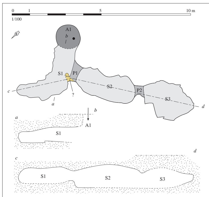
Relevé normalisé de la structure. DAO S. Bossard, d'après Giot, Le Roux, 1971, p. 140, fig. 1
