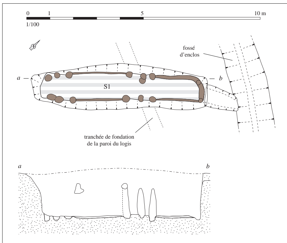
Relevé normalisé de la structure. DAO S. Bossard, d'après Menez, 2009, p. 44, fig. 36
