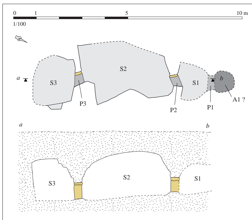
Relevé normalisé de la structure. DAO S. Bossard, d'après Le Goffic, 1993, p. 80, fig. 26
