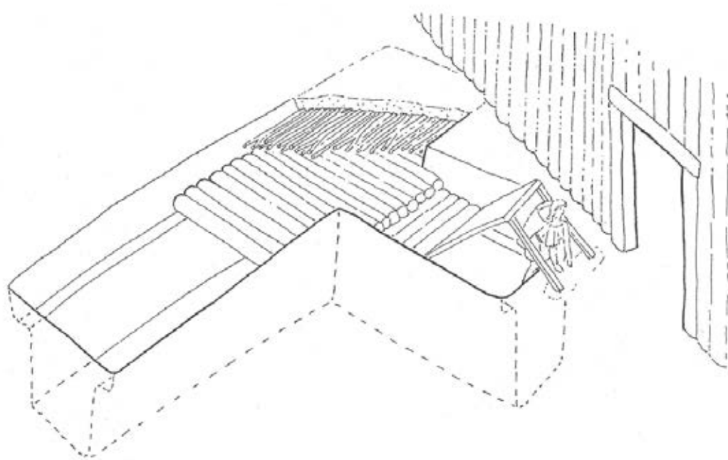
Proposition de restitution graphique de la structure, in Menez, 2009, p. 43, fig. 35
