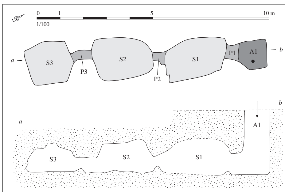
Relevé notmalisé de la structure. D'après Berthelot du Chesnay, 1906, fig. 2
