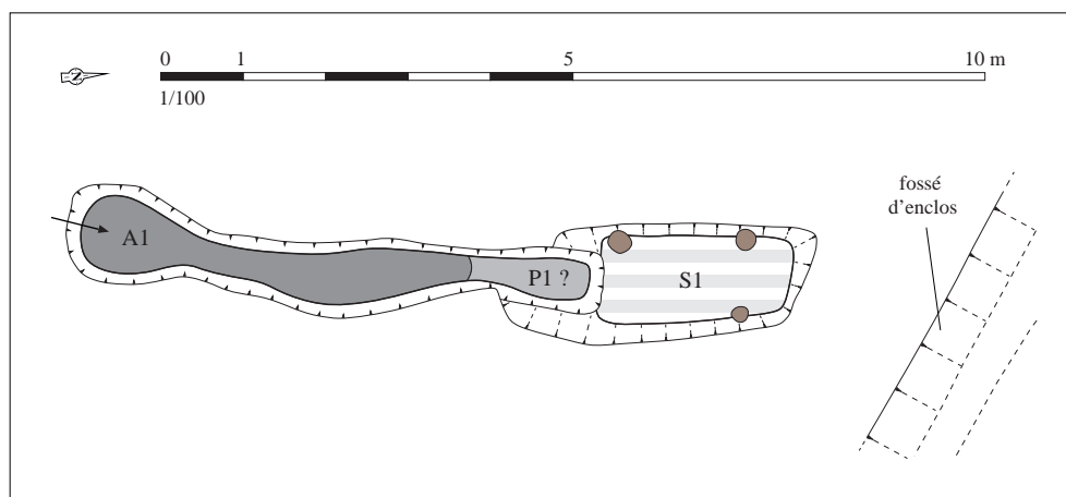
Relevé normalisé de la structure. DAO S. Bossard, d'après Menez, 2009, p. 66, fig. 58
