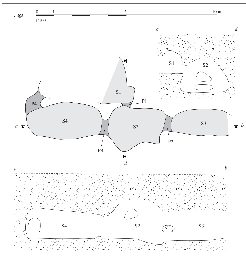
Relevé normalisé de la structure. DAO S. Bossard, d'après Provost, Le Roux, 1967, p. 122, fig. 1
