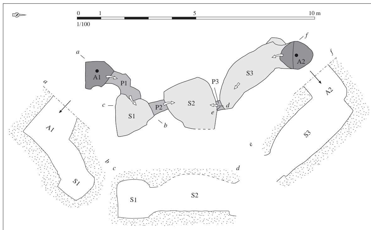
Relevé normalisé de la structure. DAO S. Bossard, d'après Moulec, 1983
