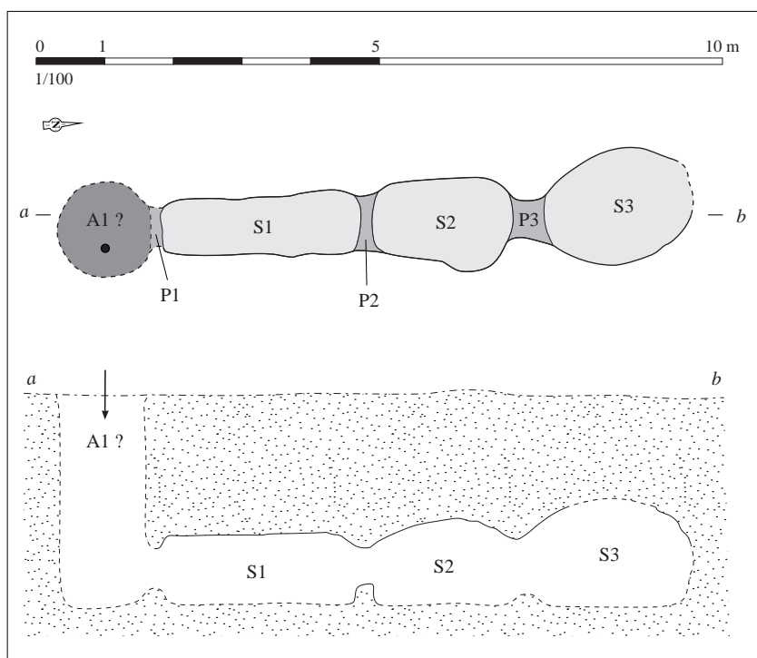
Relevé normalisé de la structure. DAO S. Bossard, d'après le Goffic, 2001, p. 82, fig. 9
