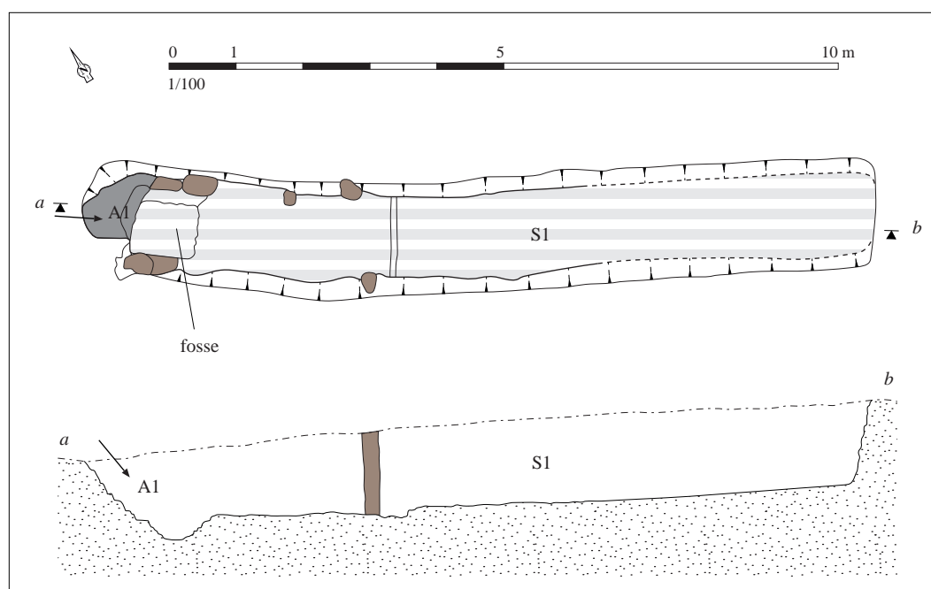
Relevé normalisé de la structure. DAO S. Bossard, d'après Menez et al., 2005, p. 15, fig. 17
