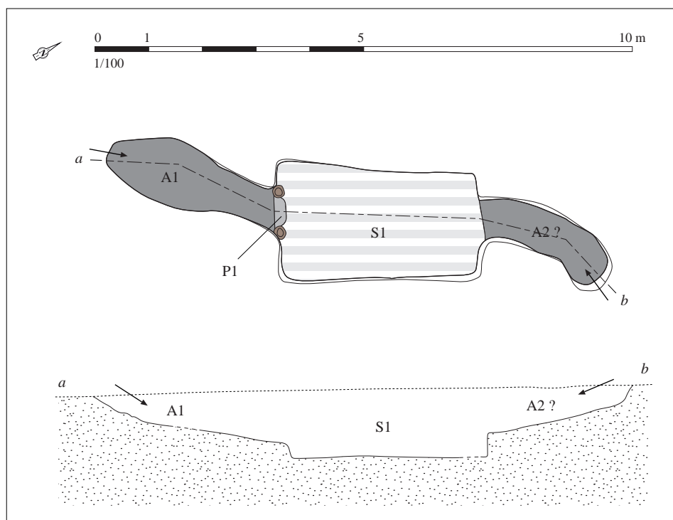
Relevé normalisé de la structure. DAO S. Bossard, d'après Le Goff (dir.), 2002, p. 505-506, fig. 363 et 364
