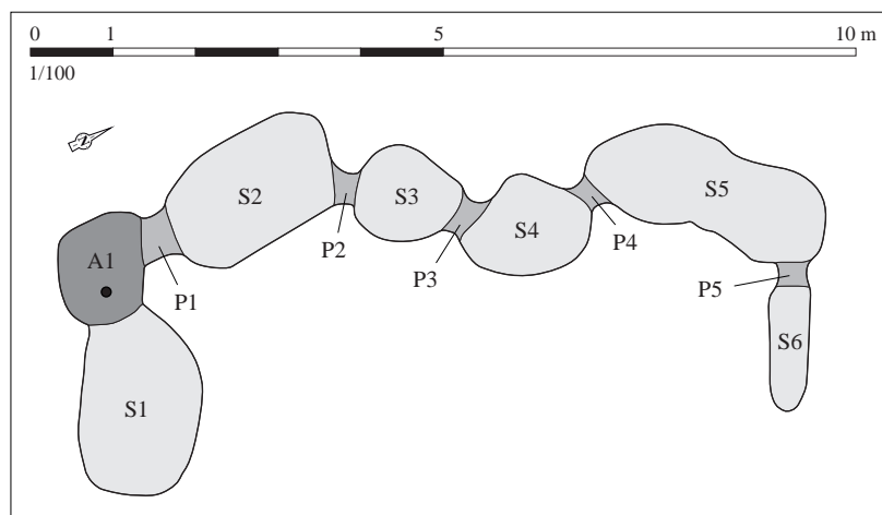
Relevé normalisé de la structure. DAO S. Bossard, d'après Tanguy, 2000, p. 155, fig. 10
