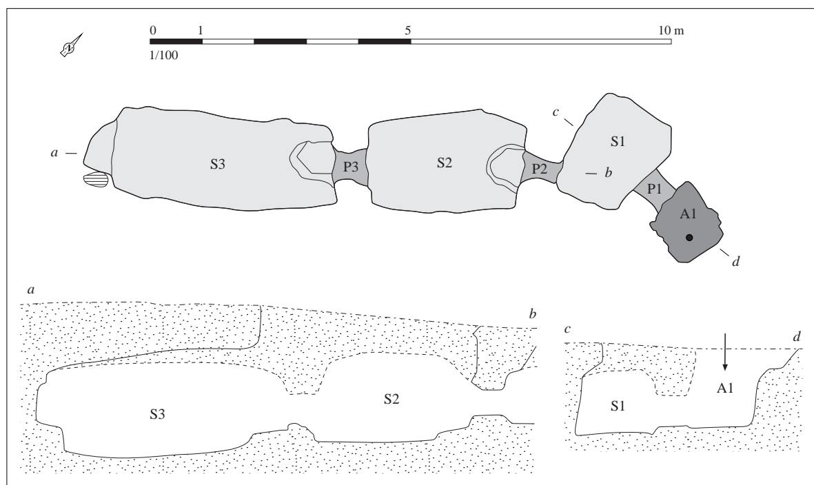
Relevé normalisé de la structure. DAO S. Bossard, d'après Hinguant, Le Goff, 1998, p. 72, fig. 14
