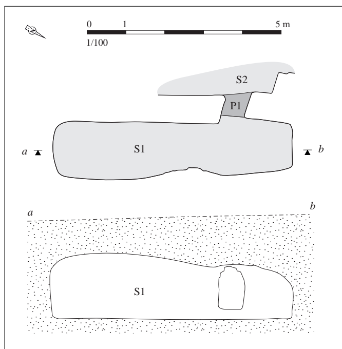
Relevé normalisé de la structure. DAO S. Bossard, d'après Lecornec, 1978, p. 120
