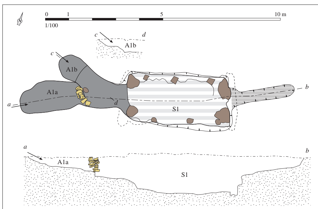
Relevé normalisé de la structure. DAO S. Bossard, d'après Demarest (dir.), 2011, pl. 48
