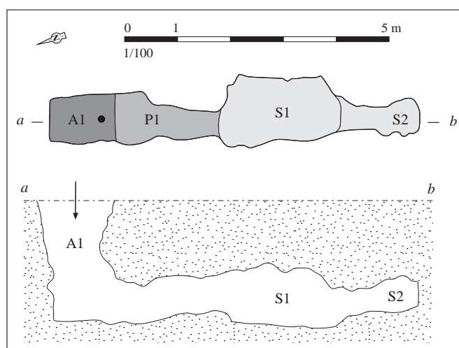
Relevé normalisé de la structure. DAO S. Bossard, d'après Tanguy, 2000, fig. 14
