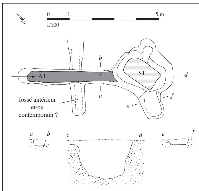
Relevé normalisé de la structure. DAO S. Bossard, d'après Nicolas, 2013, p. 87-88, fig. 72 et 73
