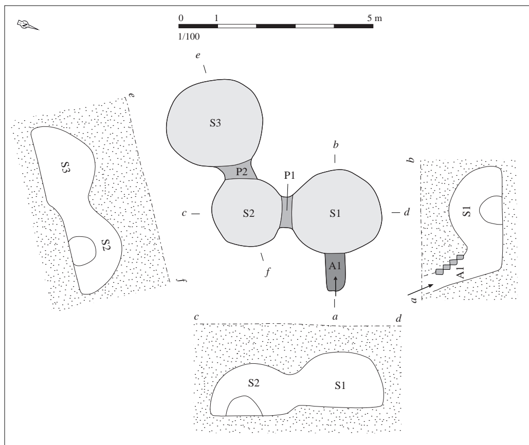
Relevé normalisé de la structure. DAO S. Bossard, d'après Sanquer, 1977, p. 3-4, et fig. 3 et 4
