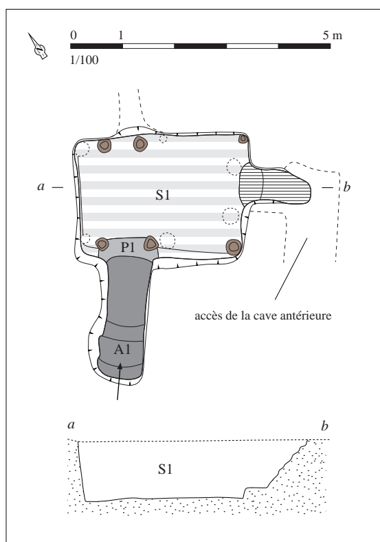
Relevé normalisé de la structure. DAO S. Bossard, d'après Le Goff (dir.), 2002, p. 517-518, fig. 370 et 371
