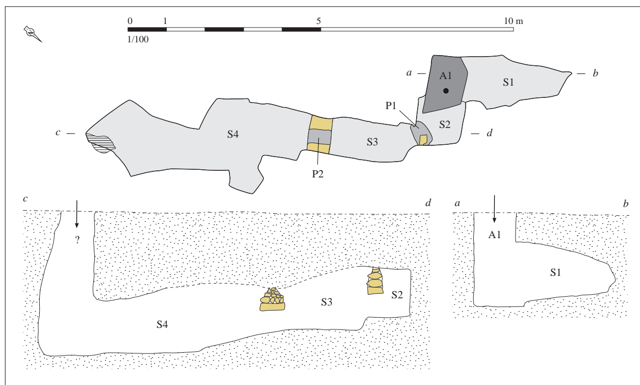
Relevé normalisé de la structure. DAO S. Bossard, d'après Bardel, 1985
