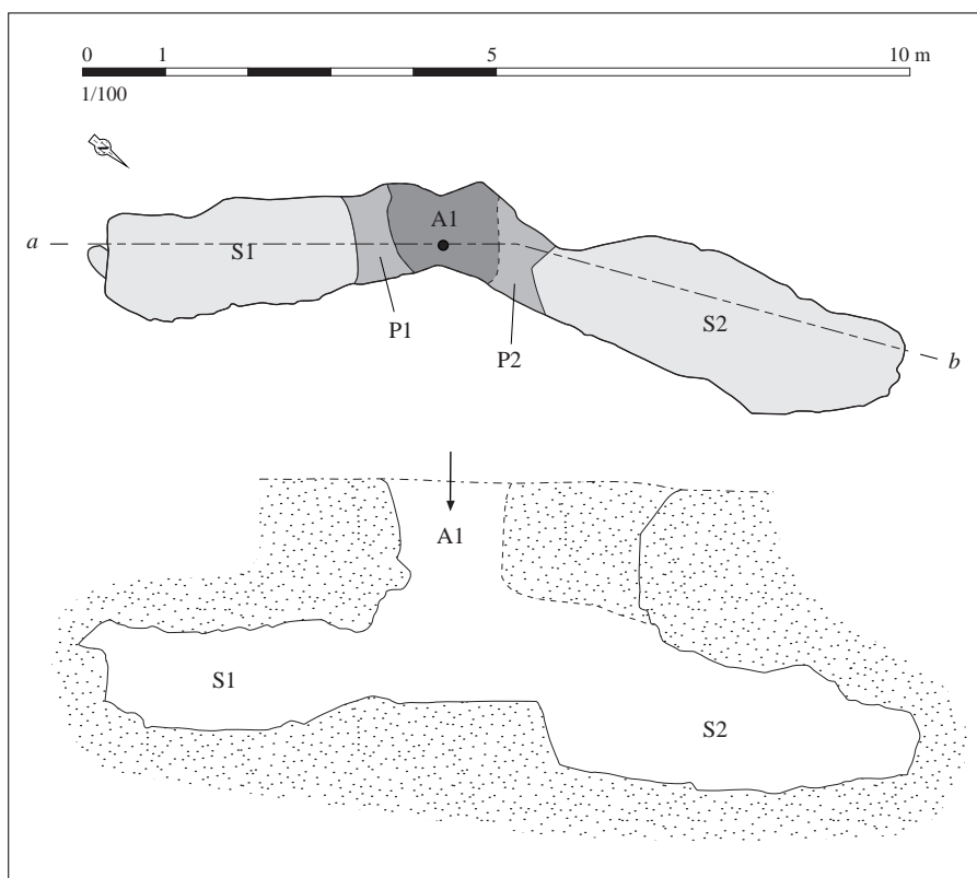
Relevé normalisé de la structure. DAO S. Bossard, d'après Le Goffic, 2003, p. 30, fig. 6
