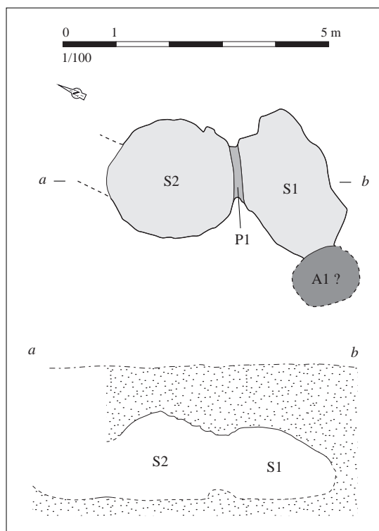
Relevé normalisé de la structure. DAO S. Bossard, d'après Le Goffic, 2003, p. 30, fig. 6
